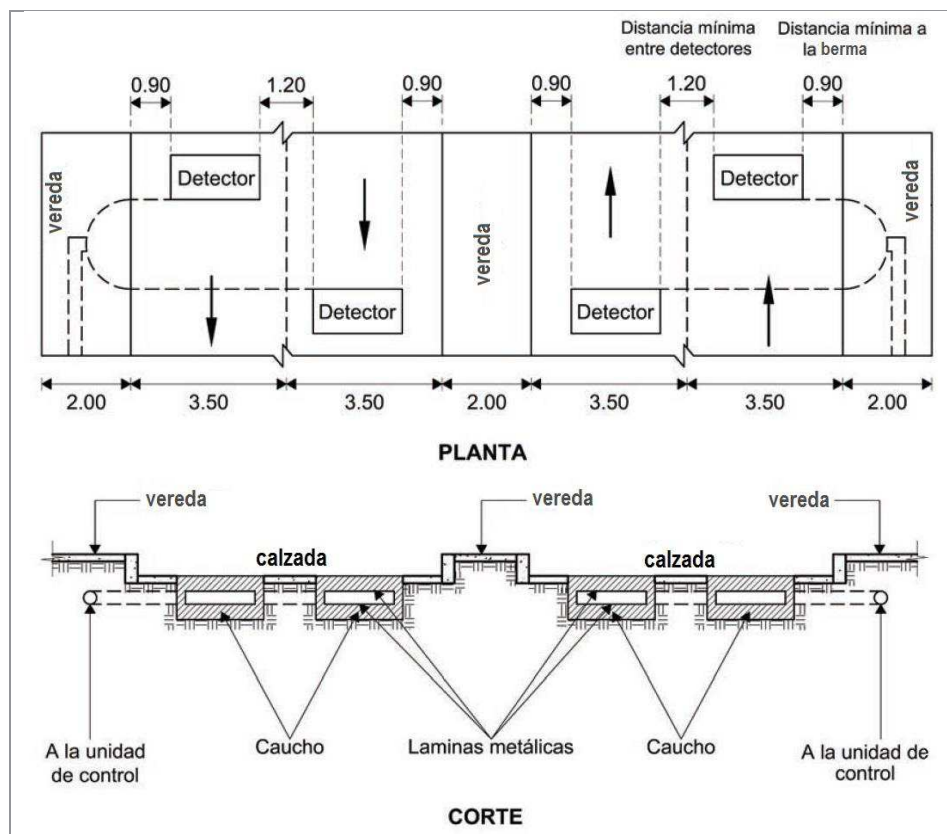
Figura 6.15 Ejemplo de ubicación transversal de detectores de presión
