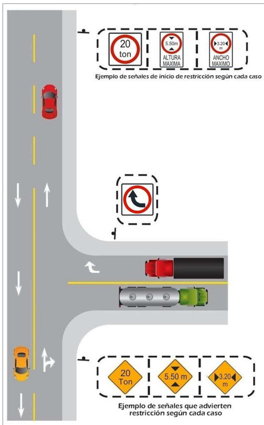
Figura 2.17 Ejemplos de señales preventivas de restricción
