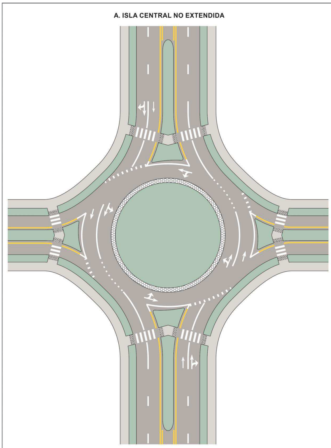
Figura 3.22 Ejemplo de demarcación para intersecciones tipo Rotonda o Glorieta de dos carriles
