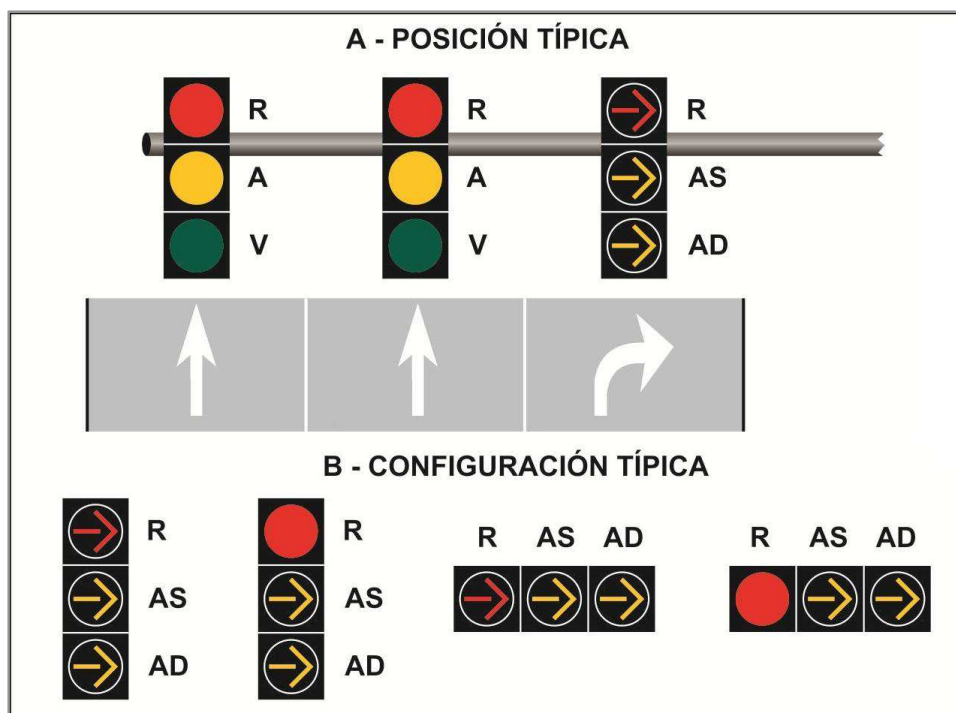
Figura 6.31 Ejemplo de disposición de indicadores de semáforos con giros a la derecha permitidos (protegidos) con ámbar destellante
