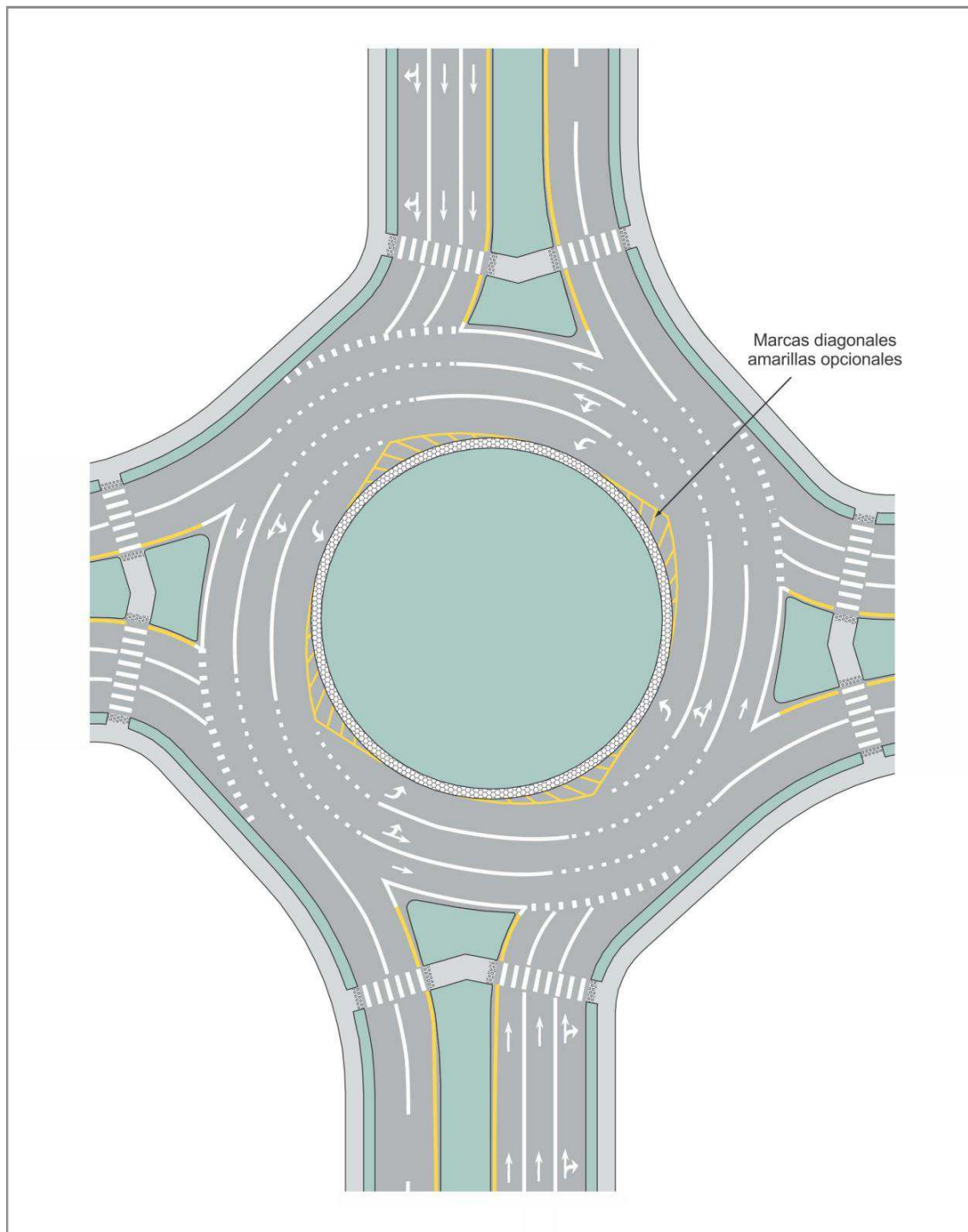
Figura 3.31 Ejemplo de demarcación para intersecciones tipo Rotonda o Glorieta de tres carriles con salidas de dos carriles
