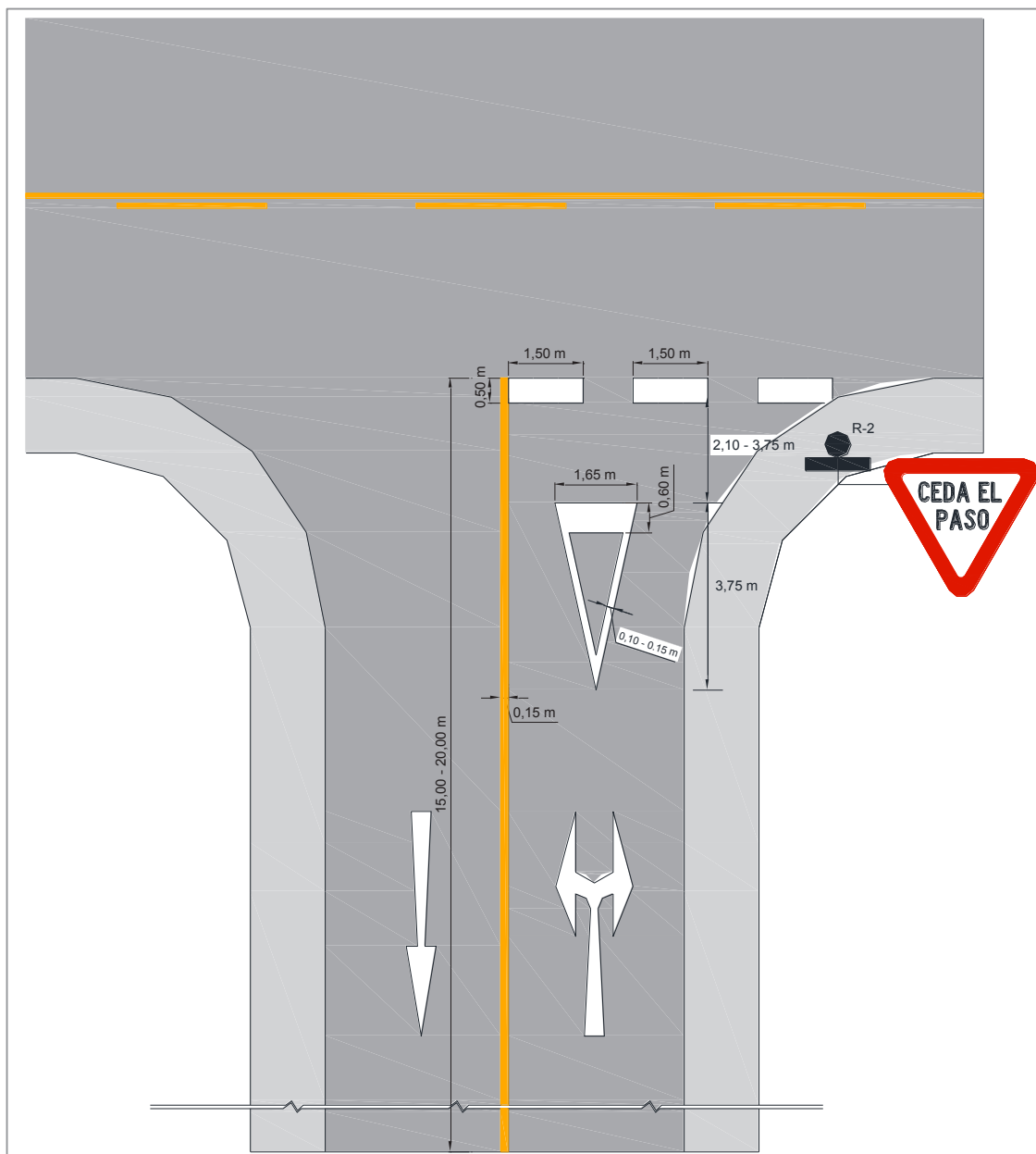
Figura 3.34 Dimensiones de demarcación "CEDA EL PASO"
