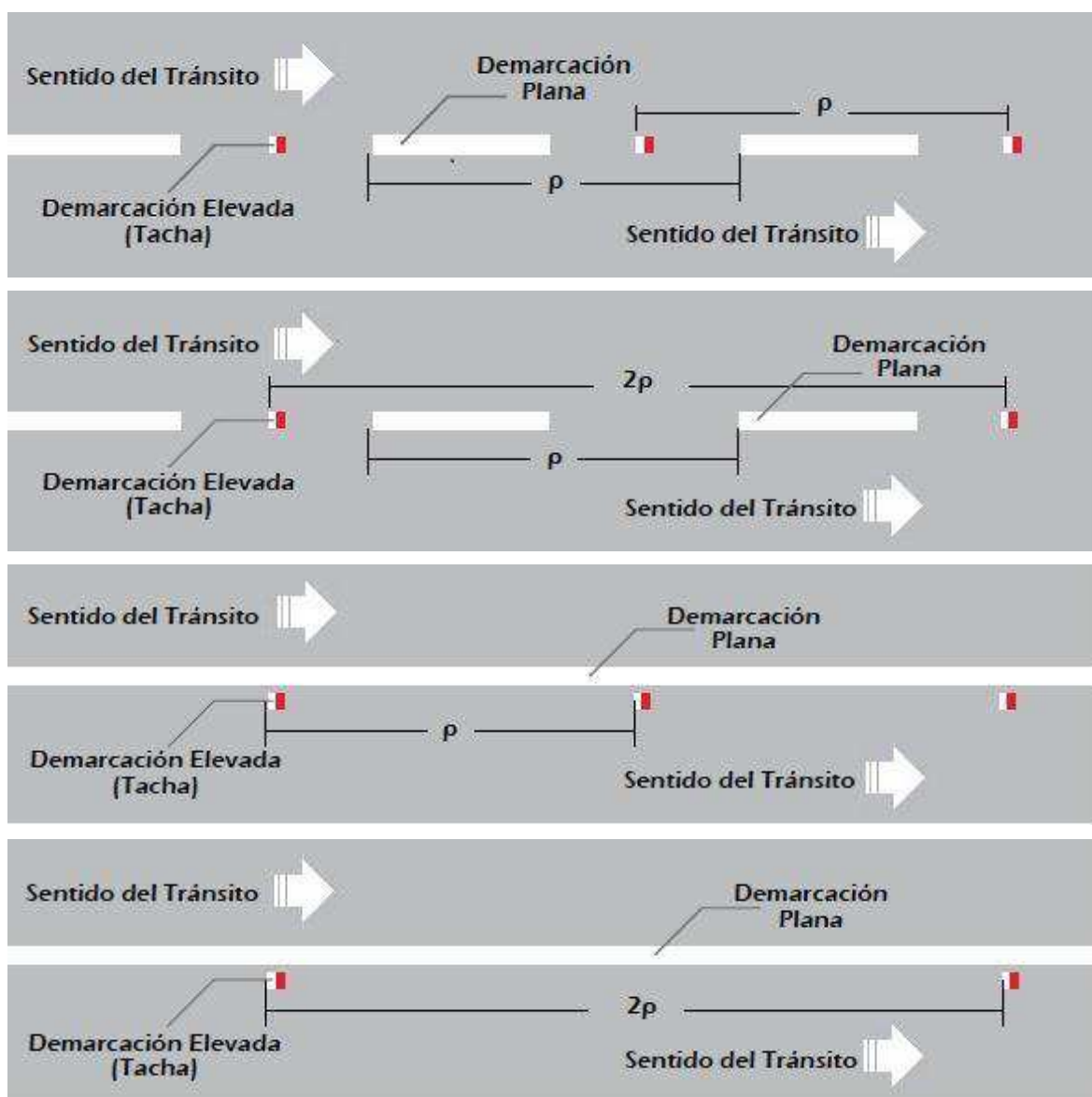
Figura 3.4 Ejemplos de línea de carril segmentada
