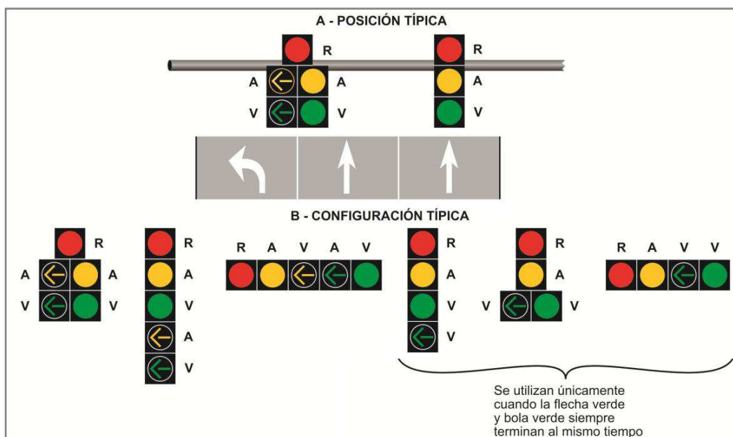
Figura 6.29 Ejemplo de disposición de indicadores de semáforos para giros a la izquierda protegidos y permitidos
