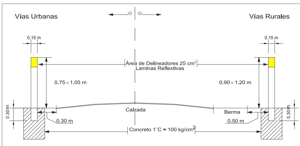
Figura 3.59 Ejemplo de altura y área mínima de material retrorreflectivo en postes delineadores
