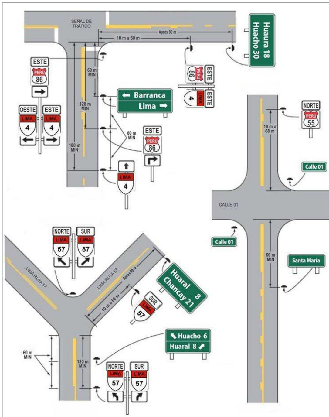
Figura 2.30 Ejemplo de conjunto de indicadores de ruta
