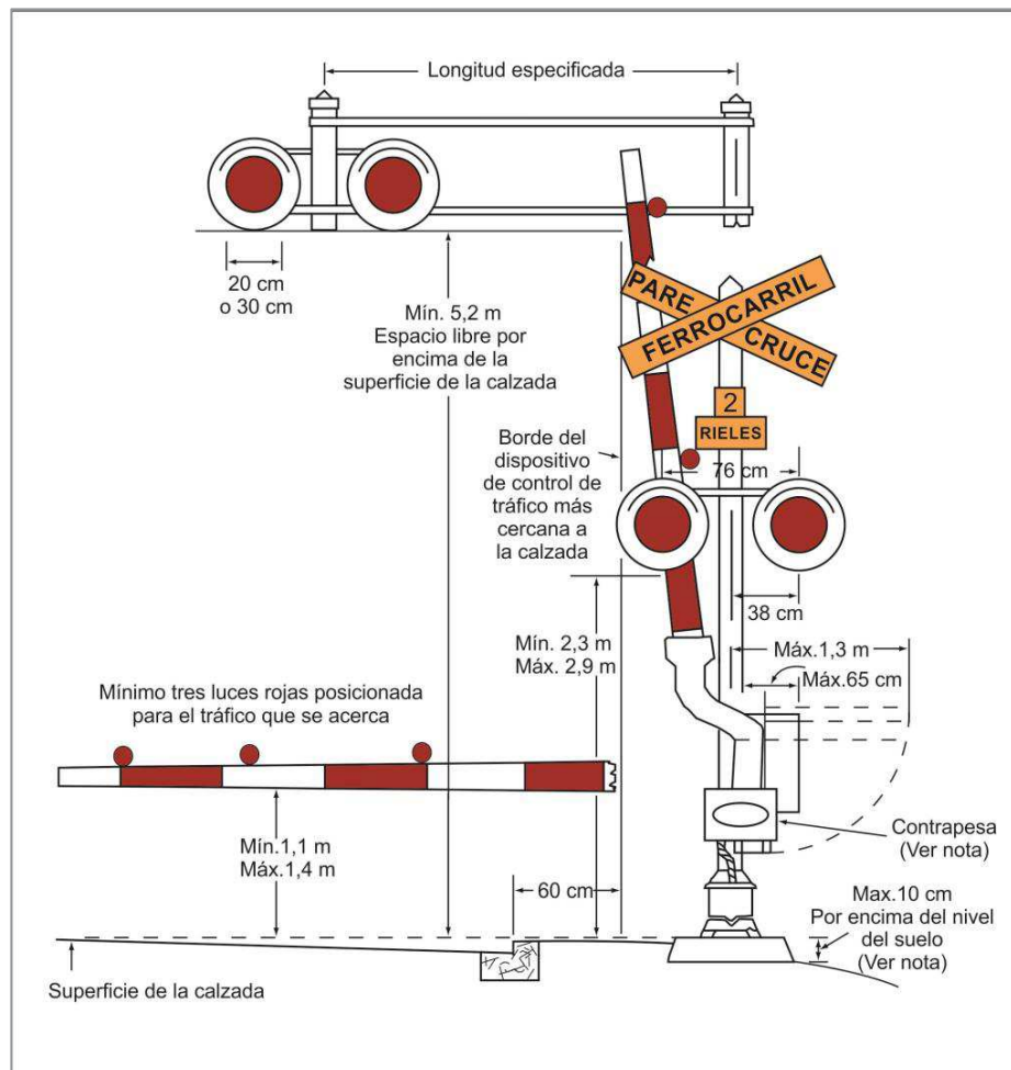
Figura 4.17 Ejemplo de un sistema de control de barreras automáticas provistas de semaforización y sensores
