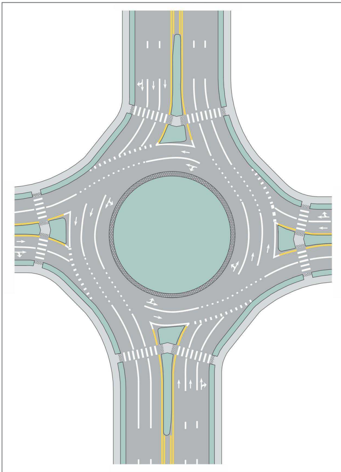
Figura 3.29 Ejemplo de demarcación para intersecciones tipo Rotonda o Glorieta de tres carriles con dos y tres carriles de entrada
