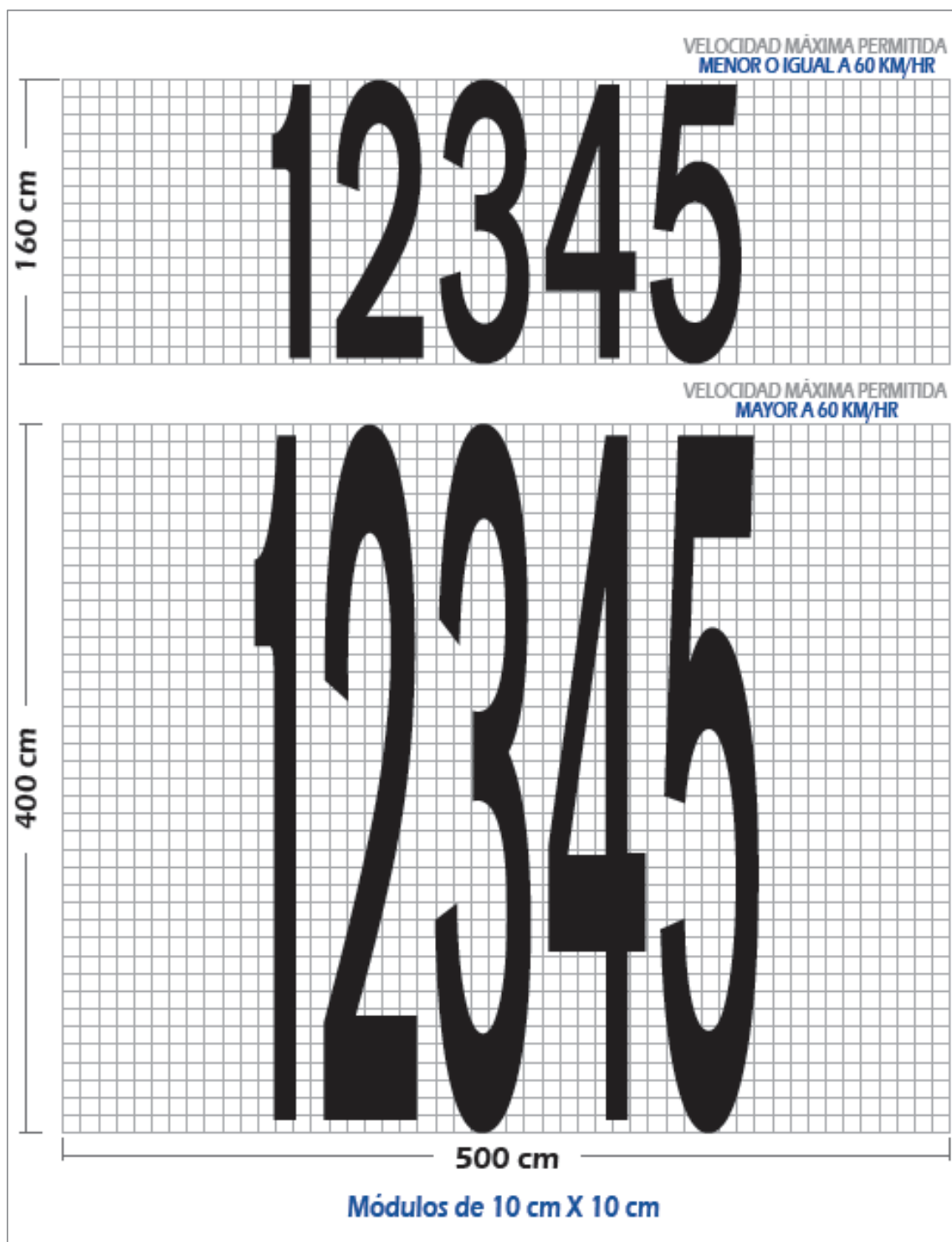
(Continua) Figura 3.53 Dimensiones de la demarcación de leyenda
