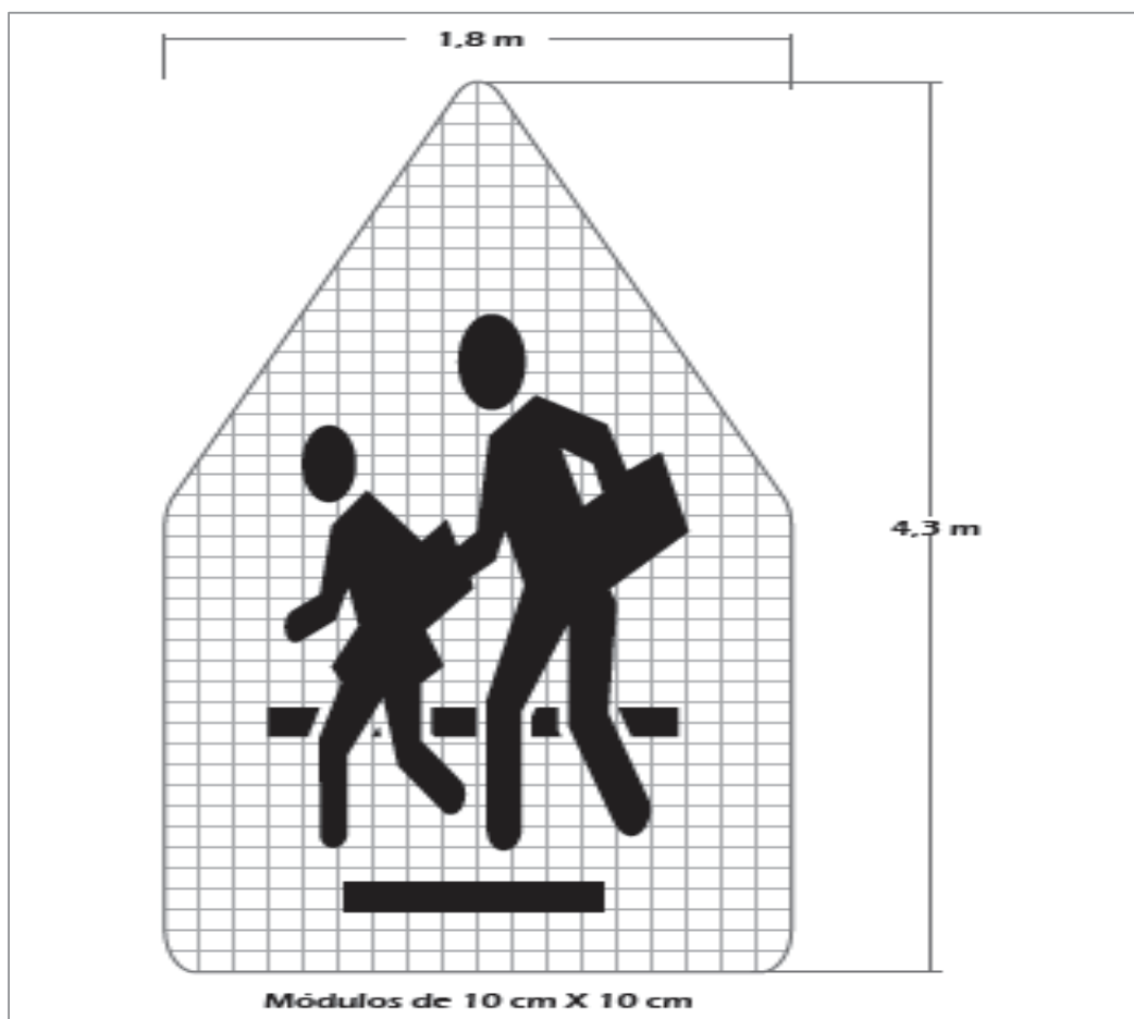
Figura 3.38 Dimensiones de demarcación “ZONA ESCOLAR”
