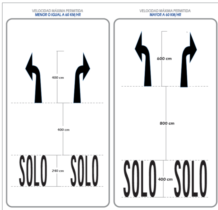
Figura 3.45 Dimensiones de flecha de giro reforzada con la palabra “SOLO”
