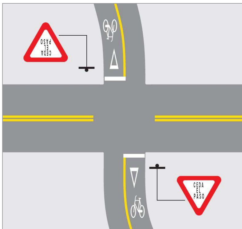
Figura 4.6 Ejemplo de aplicación de demarcación en el pavimento “CEDA EL PASO” en intersección de “CICLOVÍA” con una vía de tránsito de vehículos motorizados
