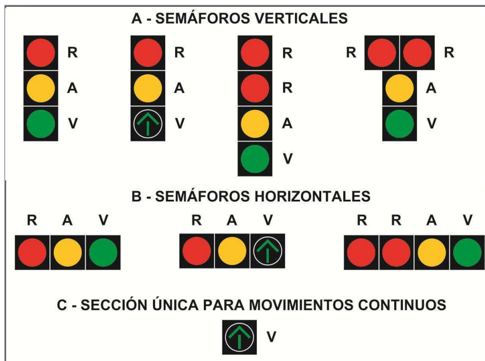
Figura 6.25 Ejemplo de disposición estándar de los indicadores de semáforos
