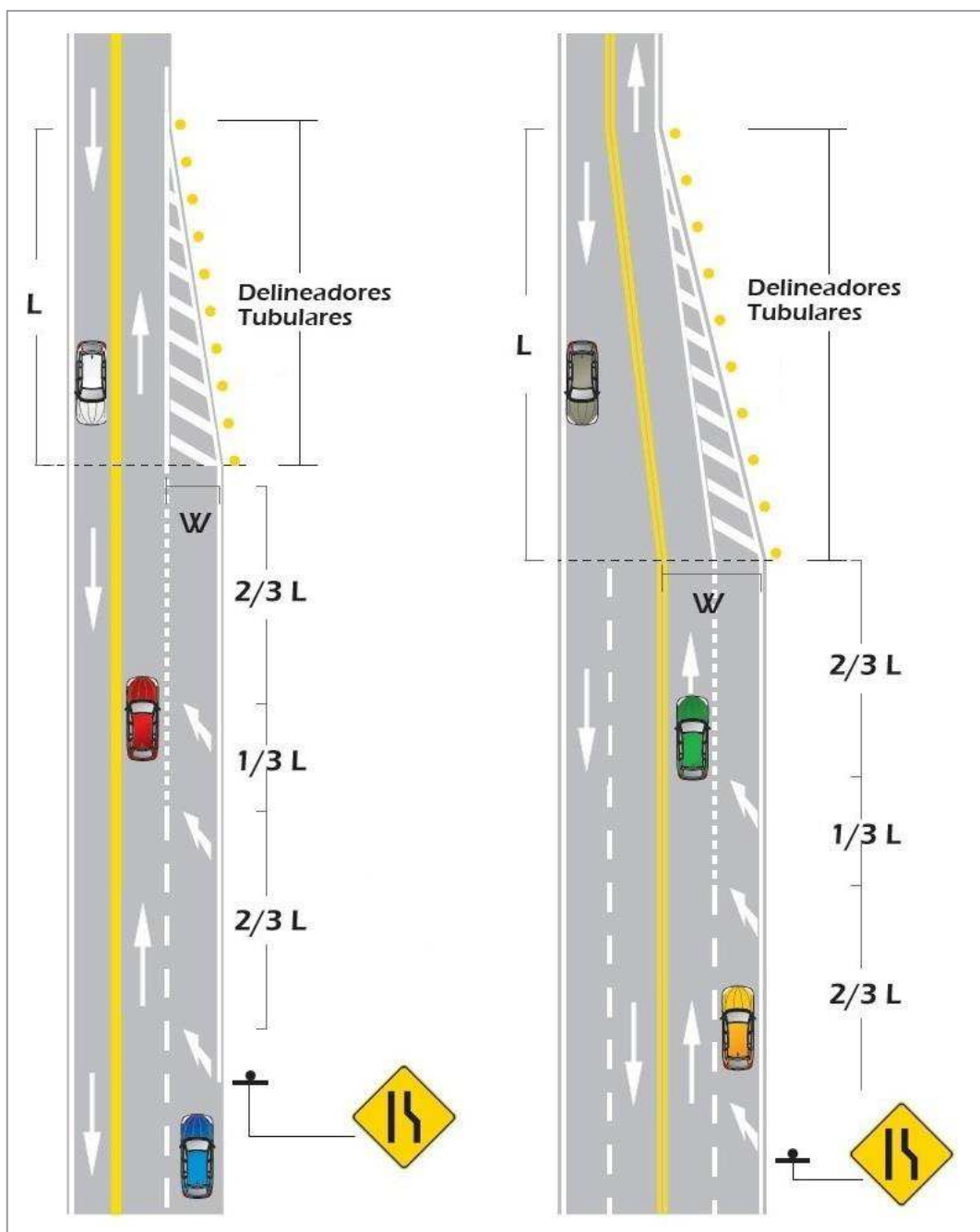
Figura 3.13 Ejemplos de Líneas de transición por reducción de carriles
