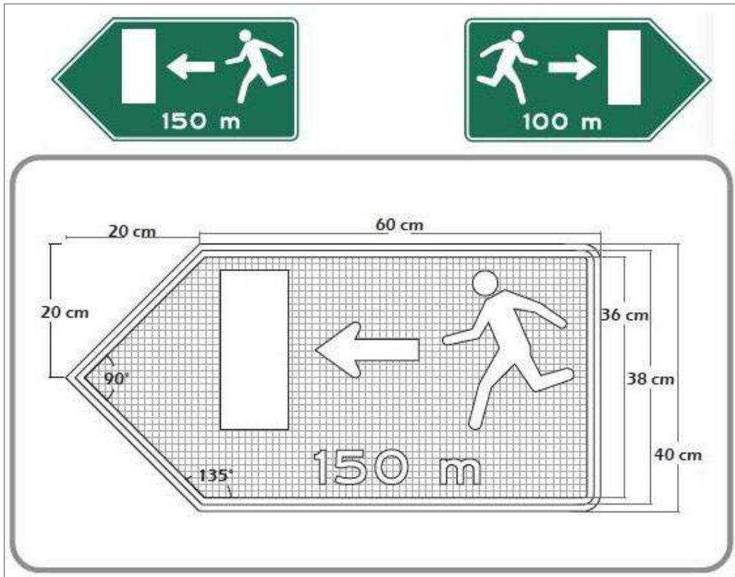
Figura 4.23 Ejemplo de señales de rutas de escape o salida de emergencia para personas, y dimensiones
