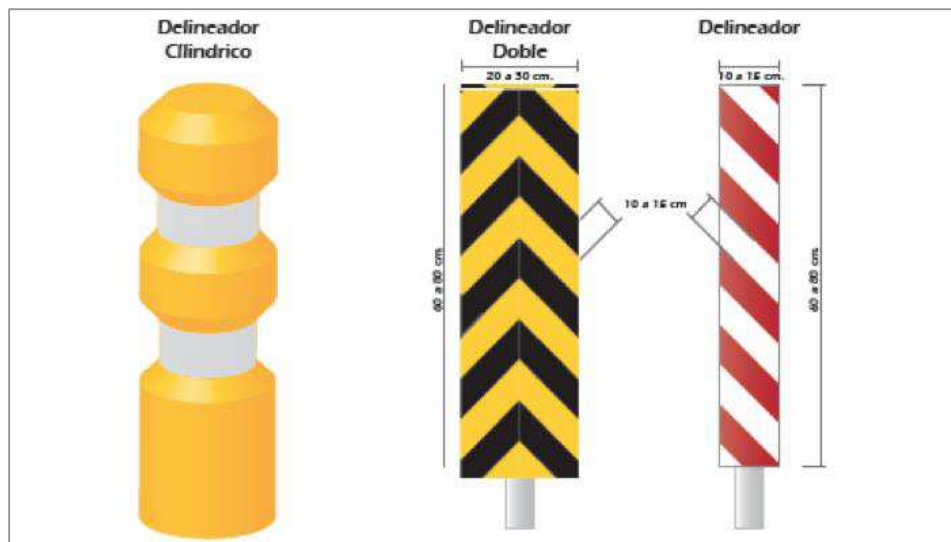
Figura 3.65 Ejemplos de tipos de delineadores “MARCADORES EN ZONAS SINGULARES”
