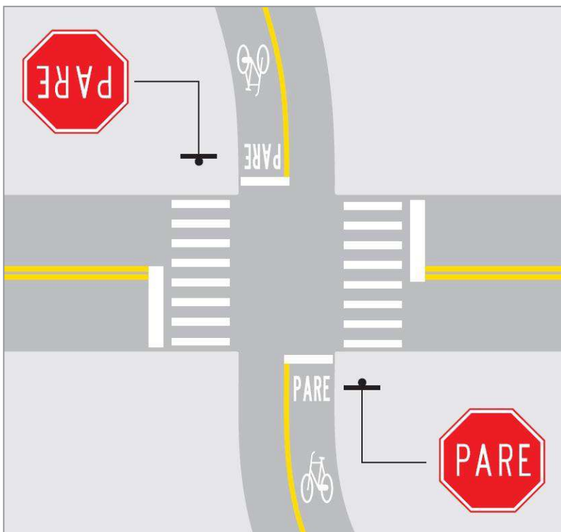
Figura 4.8 Ejemplo de aplicación de demarcación en el pavimento "PARE" en intersección de "CICLOVÍA" con una vía de tránsito de vehículos motorizados
