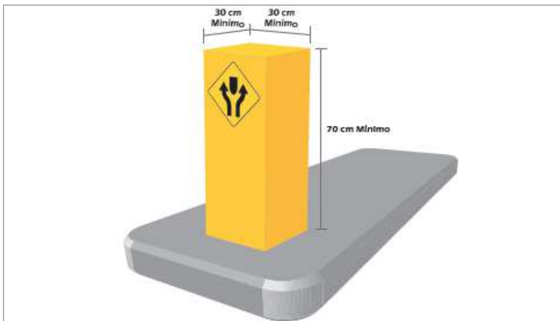
Figura 3.69 Ejemplo de demarcación de delineador tipo “Hito Luminoso”
