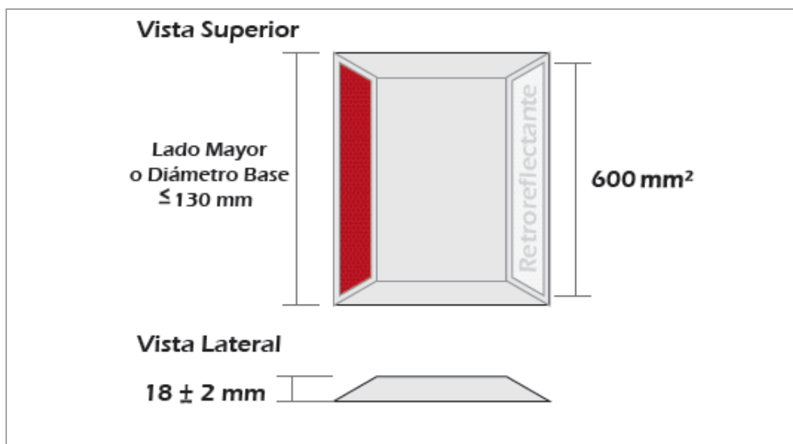
Figura 3.54 Ejemplo de Tacha retrorreflectiva u “ojo de gato”
