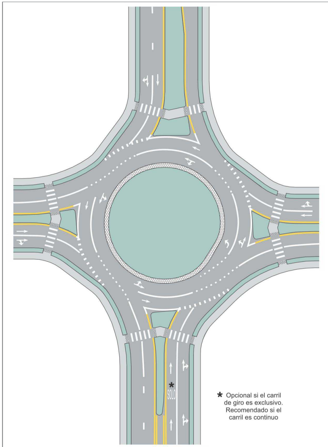
Figura 3.26 Ejemplo de demarcación para intersecciones tipo Rotonda o Glorieta de dos carriles con doble giro a la izquierda
