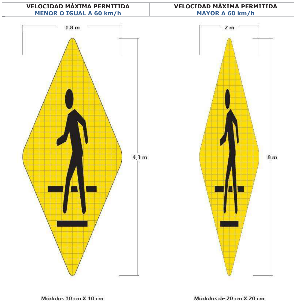
Figura 3.37 Dimensiones de demarcación (P-48) "ZONA DE PEATONES", (P-48A) "PROXIMIDAD DE CRUCE PEATONAL" y (P-48B) "UBICACIÓN DEL CRUCE PEATONAL"
