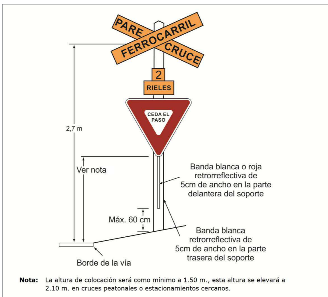
Figura 4.14 Ejemplos de la señalización vertical y dimensiones para cruces ferroviario a nivel
