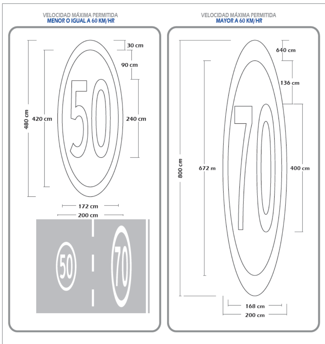
Figura 3.35 Dimensiones de demarcación “VELOCIDAD MÁXIMA PERMITIDA”
