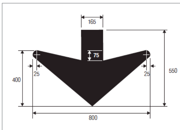
Figura 2.27 Dimensiones de flecha descendente en señales aéreas (cm)
