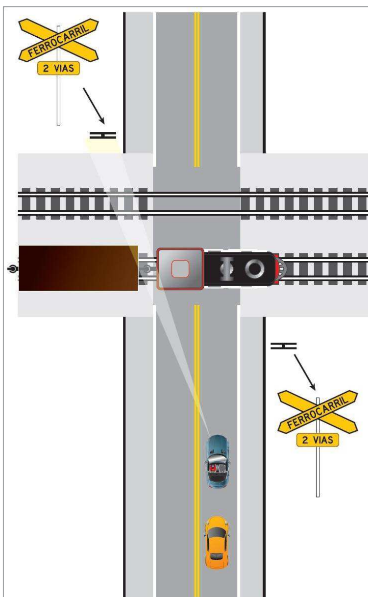
Figura 4.13 Ejemplo de señalización en cruce ferroviario a nivel.
