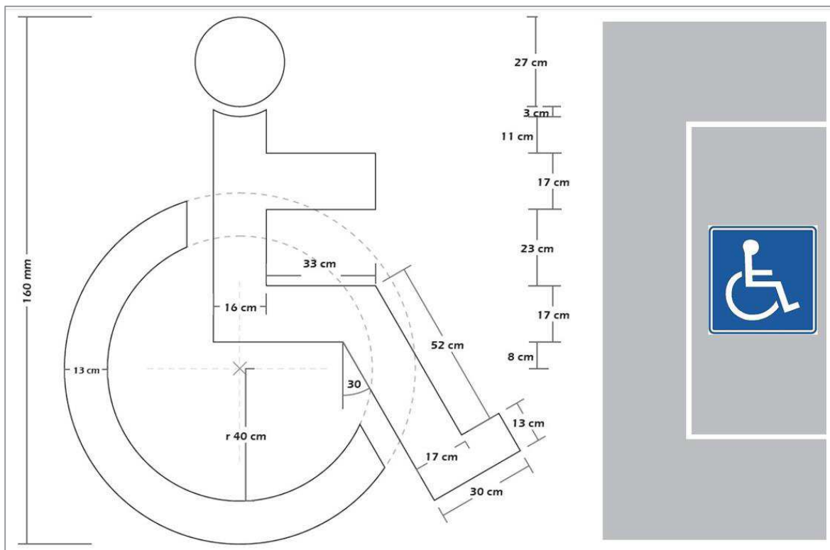
Figura 3.36 Ejemplo de demarcación y dimensiones de estacionamiento exclusivo para personas con movilidad reducida, madres gestantes y/o niños en brazos, y personas de la tercera edad
