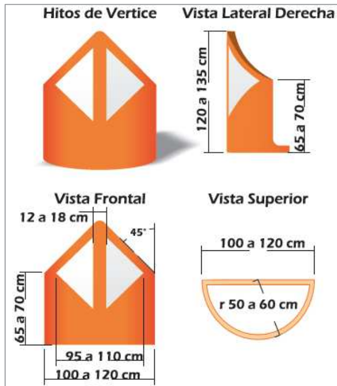
Figura 5.10 Ejemplo de hitos de vértice con dimensiones
