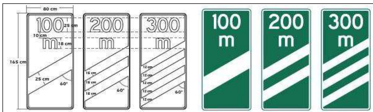
Figura 2.36 Balizas de Acercamiento
