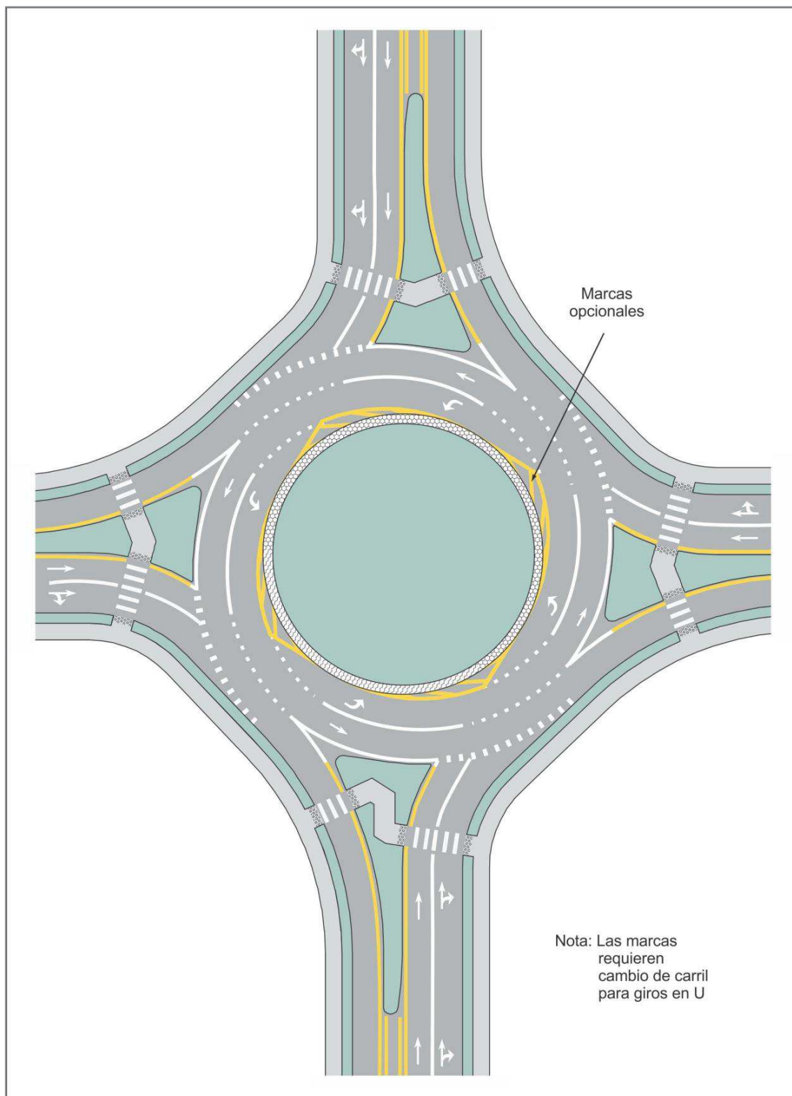
Figura 3.24 Ejemplo de demarcación para intersecciones tipo Rotonda o Glorieta de dos carriles con un carril de salida
