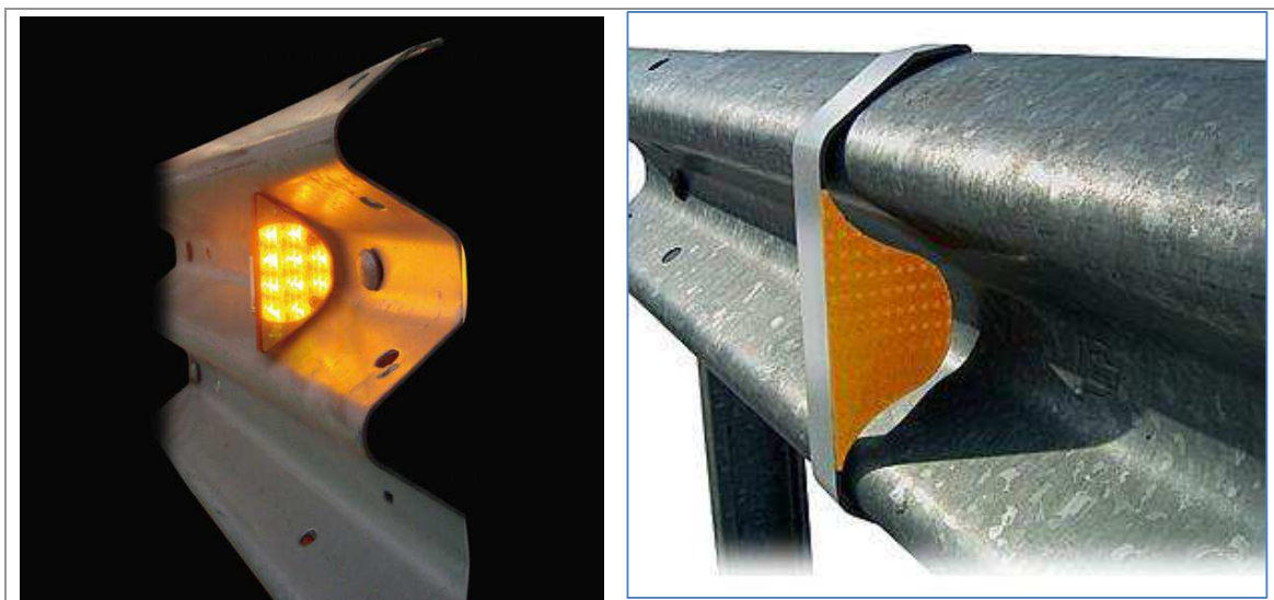
Figura 3.64 Ejemplo de ubicación de delineadores de placa “CAPTAFAROS”
