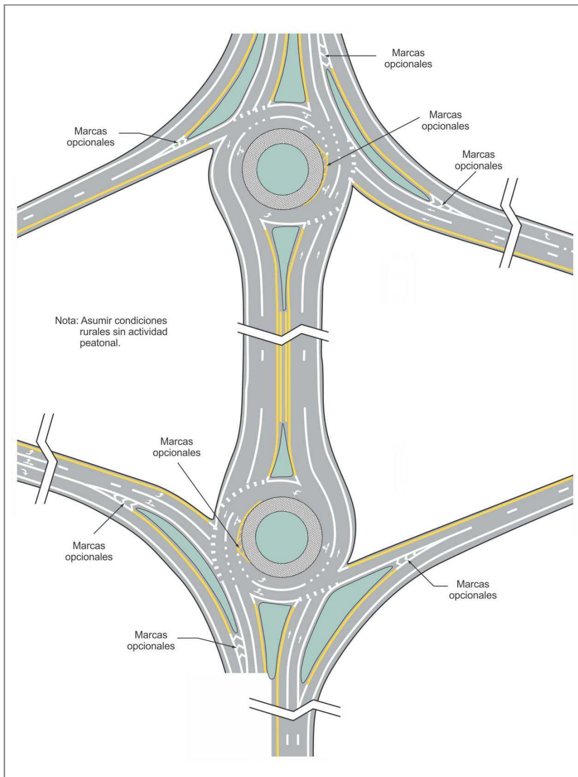
Figura 3.33 Ejemplo de demarcación para una intersecciones tipo diamante con rotondas o glorietas en los terminales de las rampas
