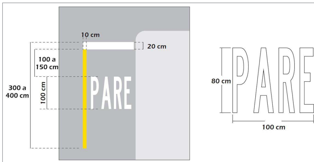
Figura 4.9 Ejemplo de dimensiones de demarcación en el pavimento "PARE" en intersección de "CICLOVÍA" con una vía de tránsito de vehículos motorizados.
