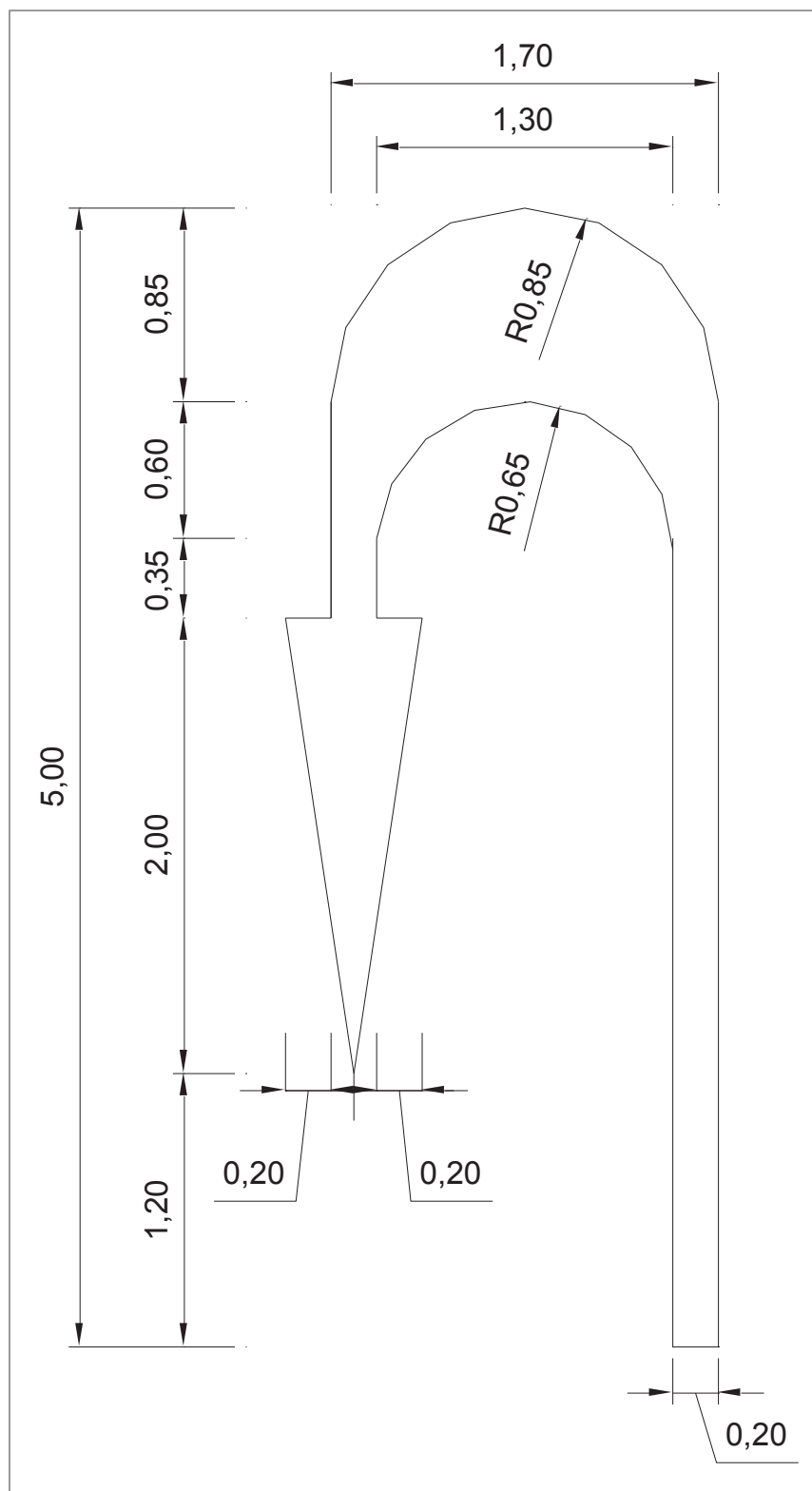
Figura 3.48 Dimensiones de flecha de giro en "U"
