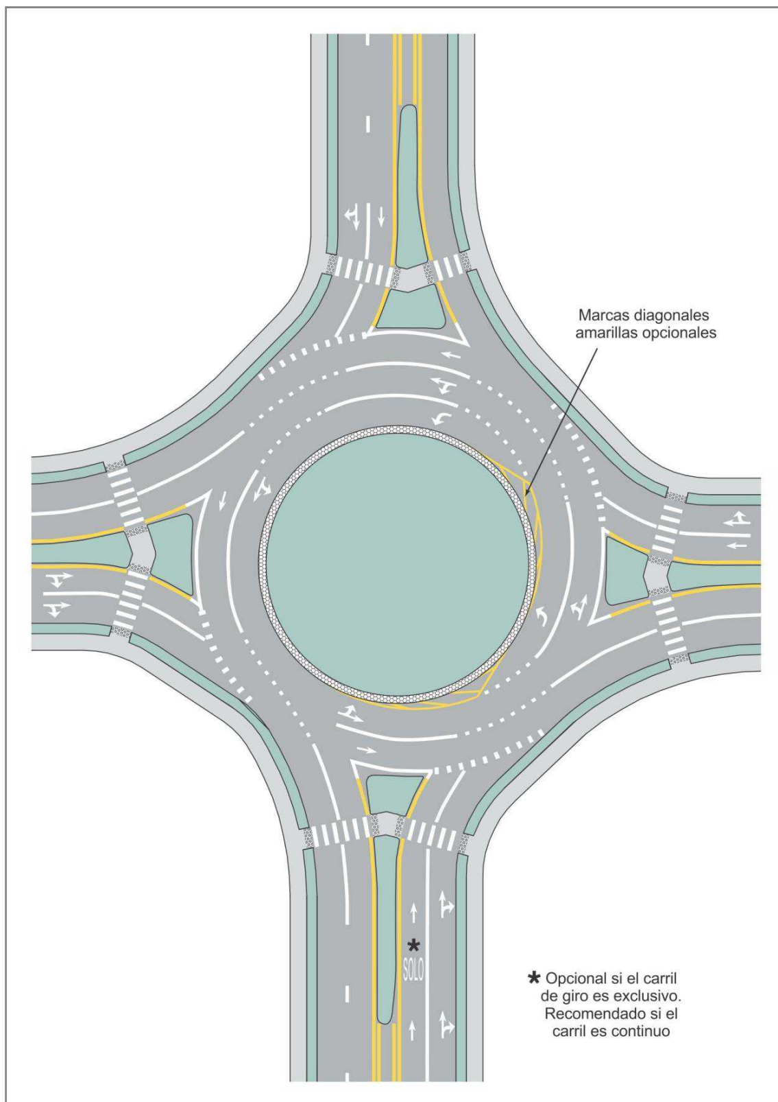
Figura 3.28 Ejemplo de demarcación para intersecciones tipo Rotonda o Glorieta de dos carriles con doble giro consecutivo a la izquierda
