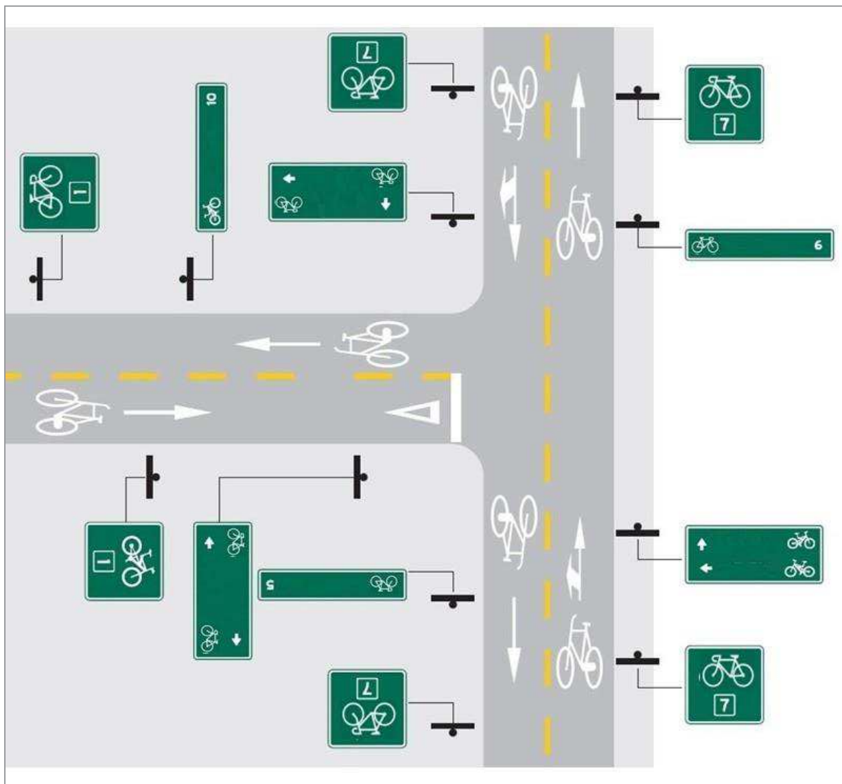
Figura 4.4 Ejemplo de aplicación de una señalización en una intersección de "CICLOVÍAS".
