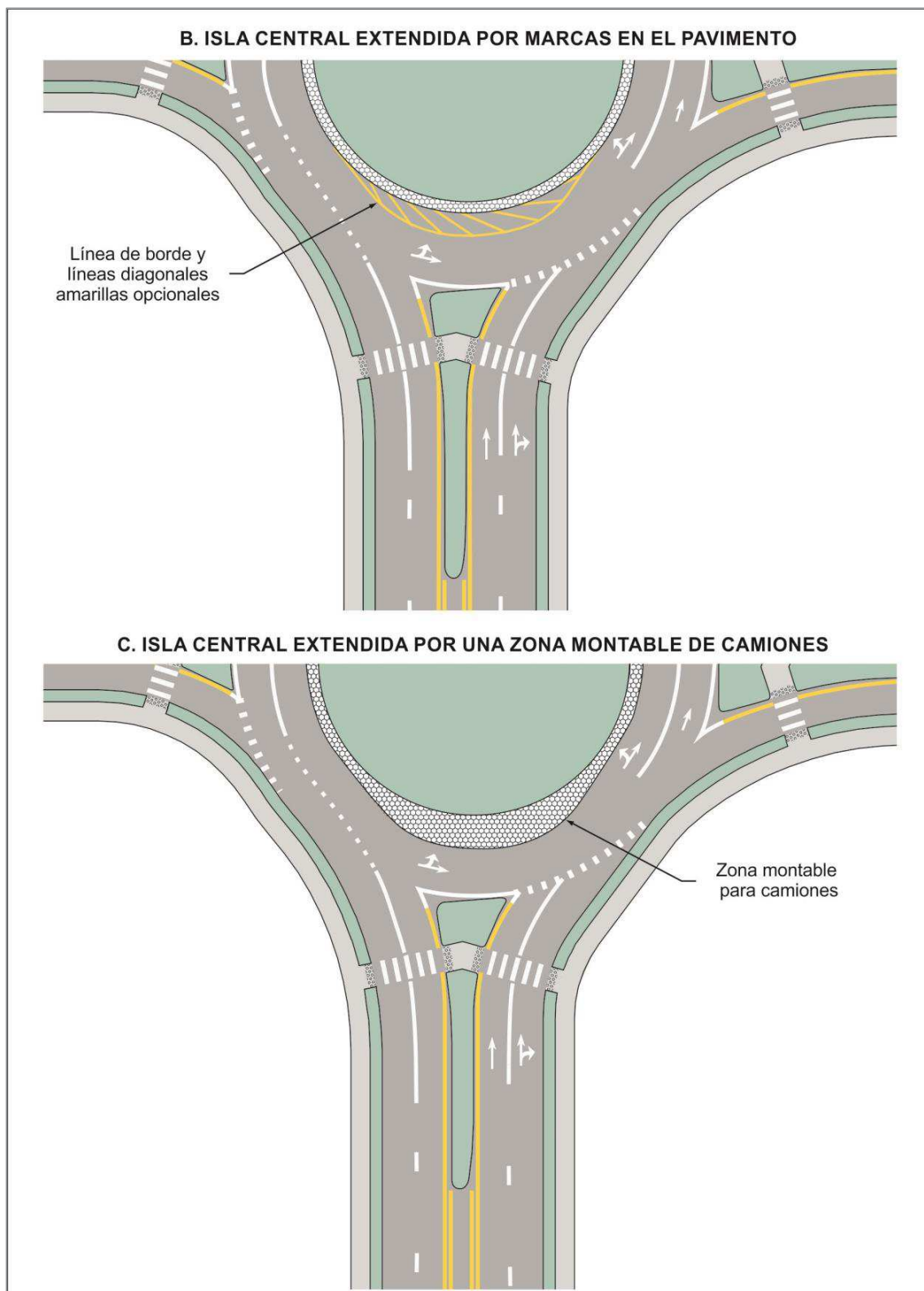
Figura 3.23 Ejemplo de demarcación para intersecciones tipo Rotonda o Glorieta de dos carriles con uno o dos carriles de circulación
