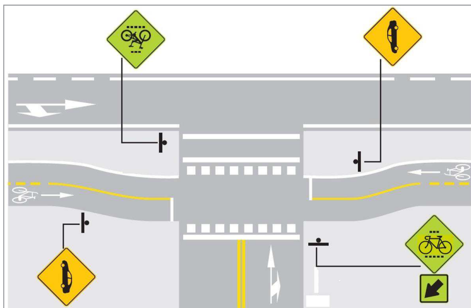
Figura 4.5 Ejemplo de aplicación de demarcación en el pavimento y señalización vertical de “CICLOVÍA” en una intersección vial
