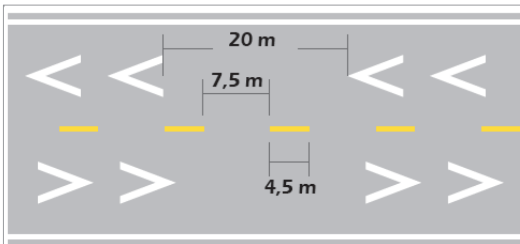
Figura 3.39 Ejemplo de demarcación de “DISTANCIADORES”
