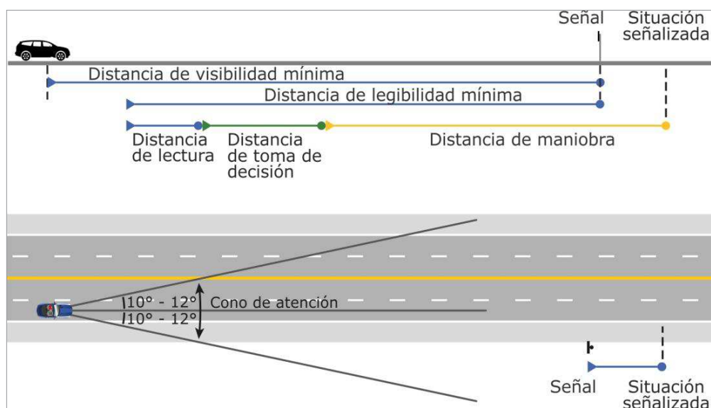
Figura 2.4 Ubicación Longitudinal y Distancias de Lectura
