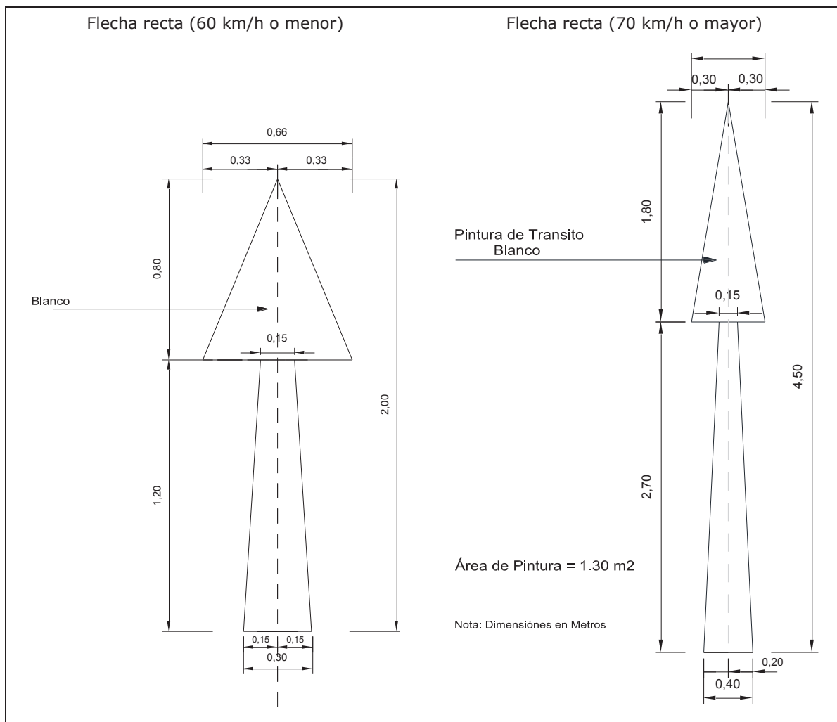
Figura 3.43 Dimensiones de flecha recta
