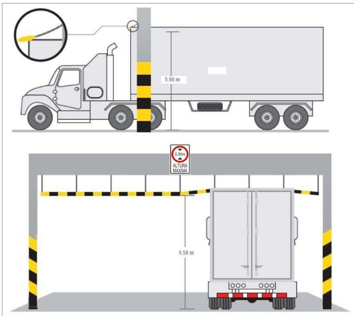
Figura 4.19 Ejemplo de un pórtico que advierte al Conductor sobre la proximidad de un túnel y la altura máxima permitida (GALIBO)
