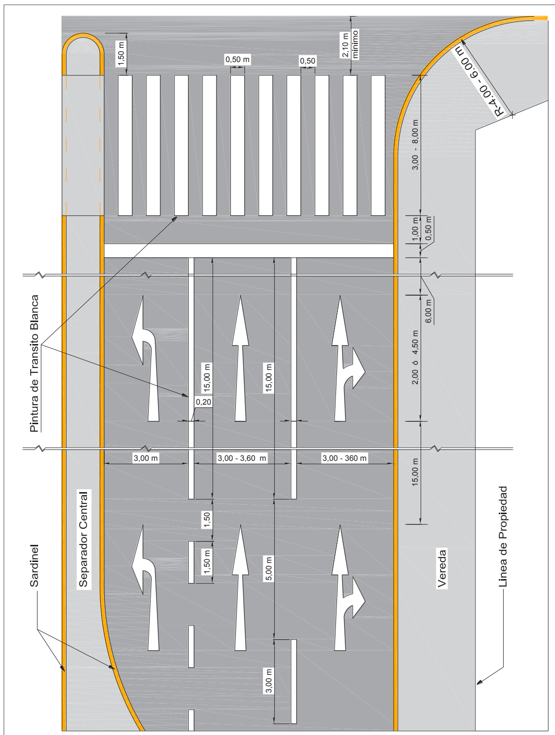
(Continua) Figura 3.14 Ejemplos de demarcación de línea de pare con dimensiones
