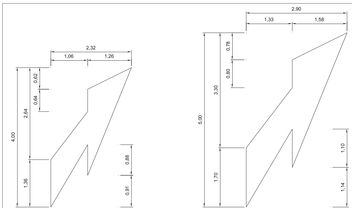
Figura 3.51 Dimensiones de flecha incorporación a carriles exclusivos
