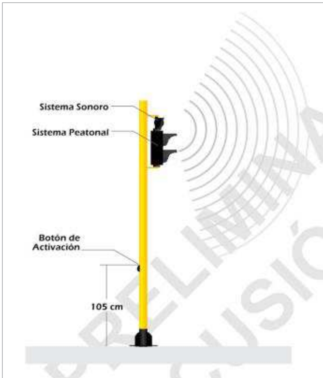
Figura 6.23 Ejemplo de un semáforo peatonal donde se indica la localización de las ondas sonoras y el dispositivo manual de activación
