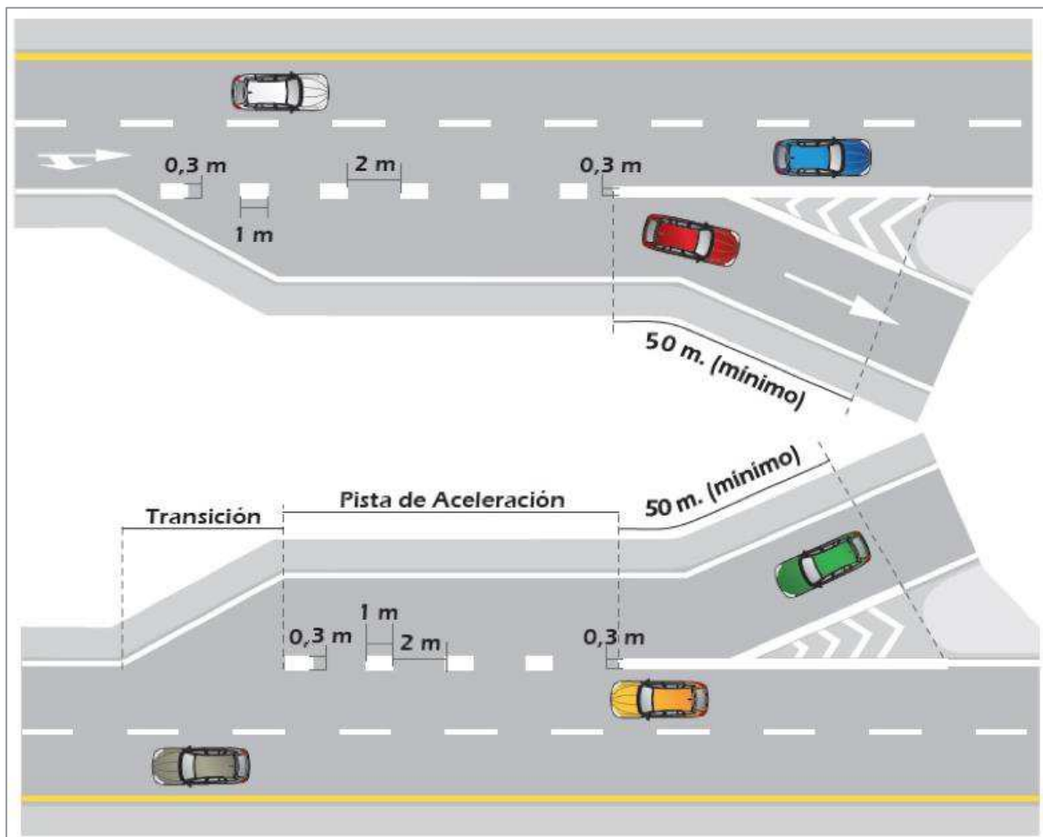
(Continua) Figura 3.3 Ejemplos de línea de borde de calzada o superficie de rodadura
