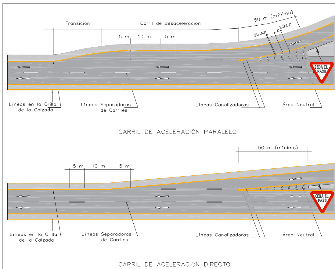
(Continua) Figura 3.12 Ejemplos de líneas demarcadoras de entradas y salidas
