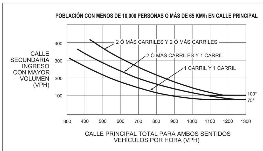
Figura 6.19: Se utiliza en función a la velocidad de la vía principal y población en zona urbana
