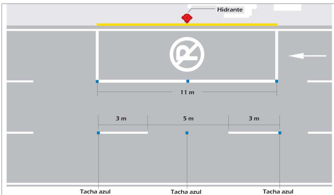
Figura 3.41 Ejemplo de demarcación de ubicación de Grifos Contra Incendios
