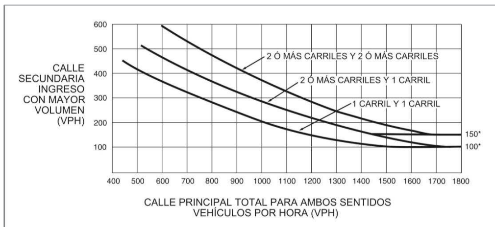
Figura 6.18 Grafico para combinación de carriles para hora punta
