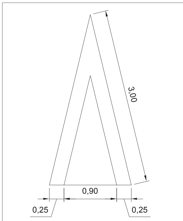
Figura 3.40 Dimensiones de demarcación de "DISTANCIADORES"
