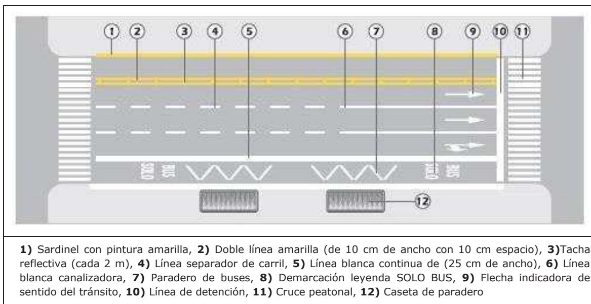
Figura 3.18 Ejemplo de demarcación de paraderos de buses
