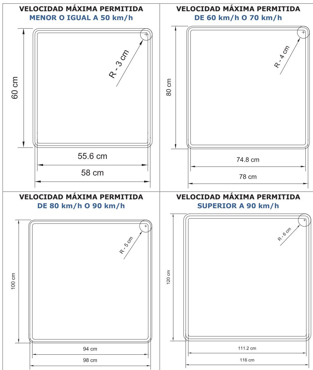
Figura 2.46 Dimensiones de placas de Señales Informativas de Servicios Generales
