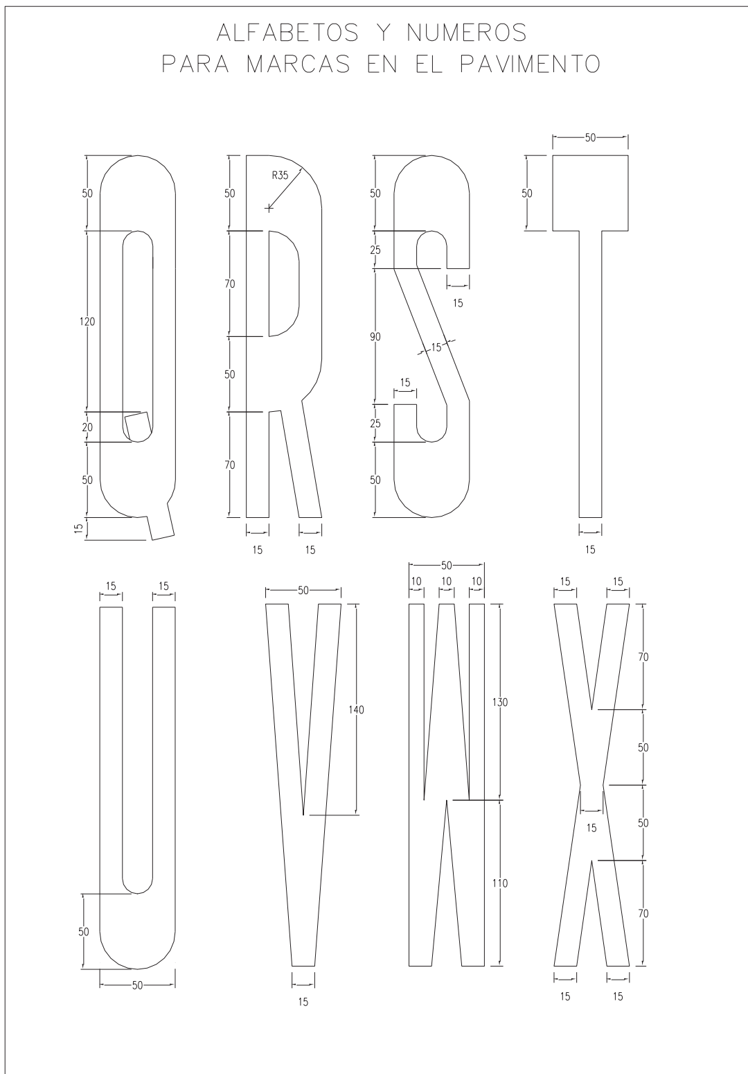
(Continua) Figura 3.53 Dimensiones de la demarcación de leyenda
