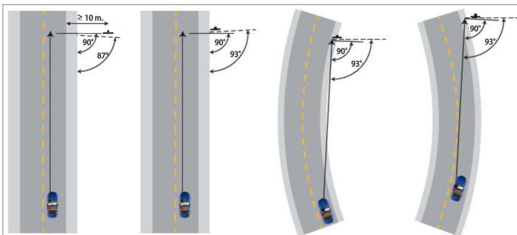
Figura 2.6 Ejemplo de Orientación de la Señal
