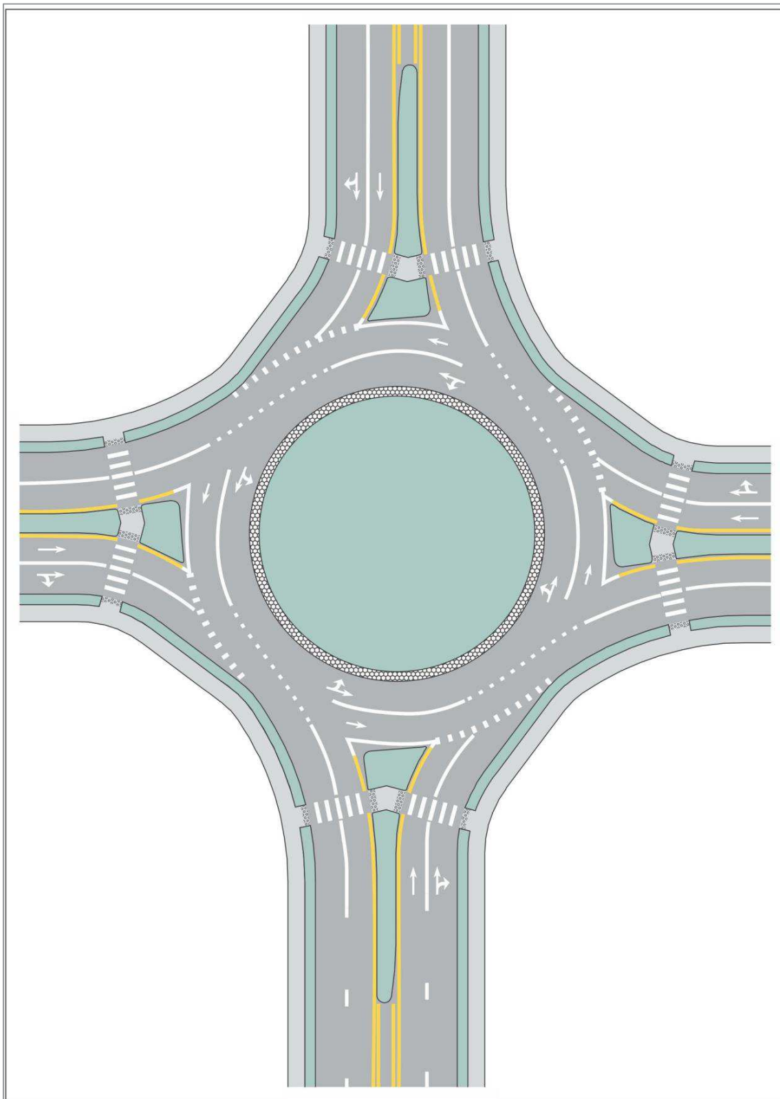
Figura 3.25 Ejemplo de demarcación para intersecciones tipo Rotonda o Glorieta de dos carriles con dos carriles de salida
