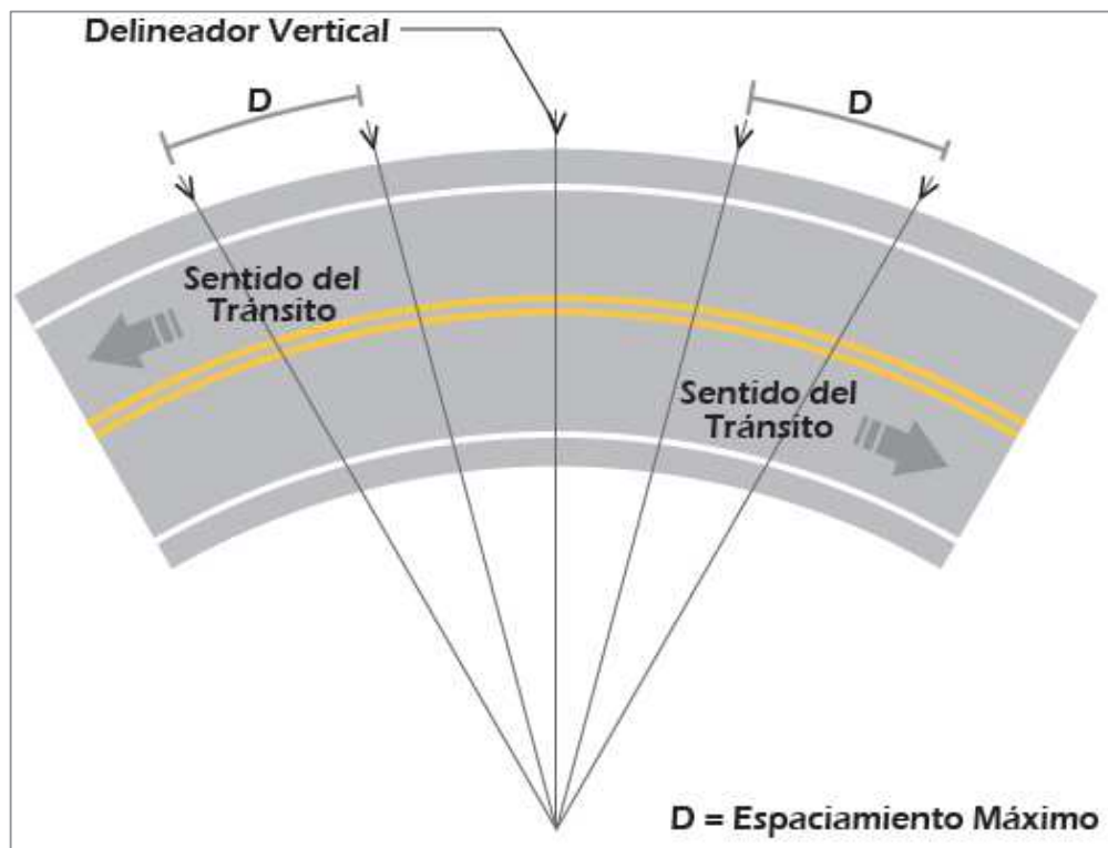
Figura 3.60 Ejemplo esquemático de ubicación de postes delineadores en curva horizontal
