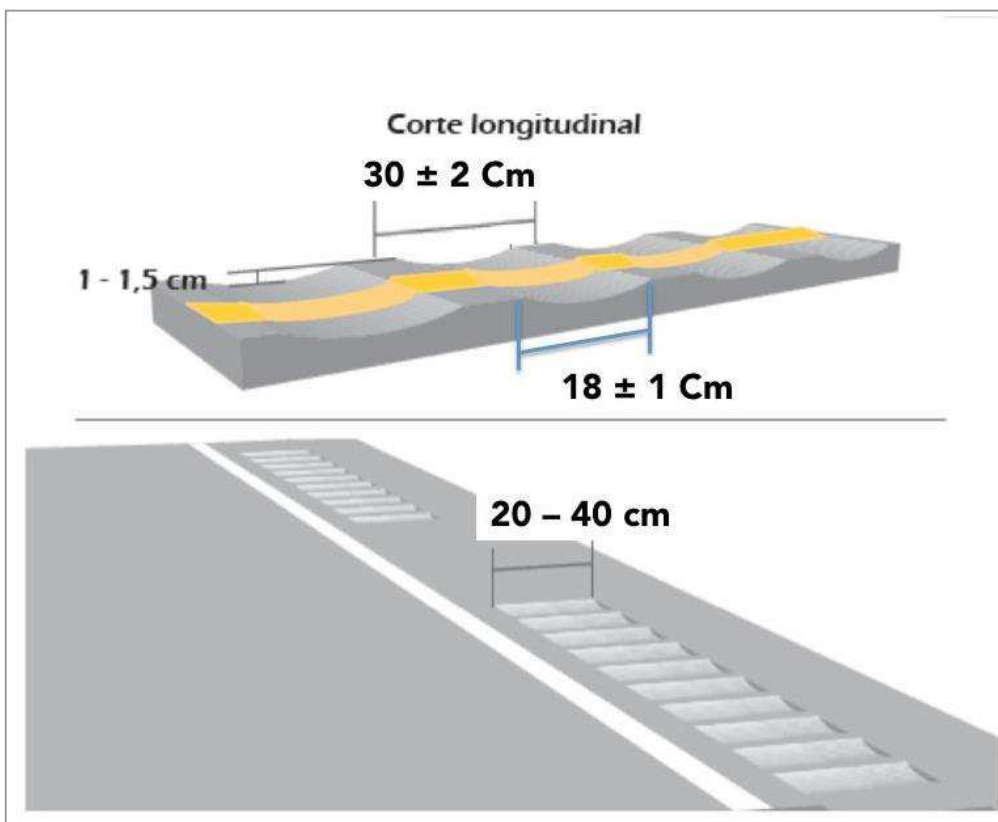
Figura 3.57 Ejemplo de demarcación bajo relieve
