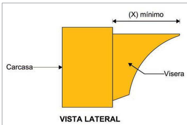
Figura 6.11 Ejemplo de visera de semáforo
