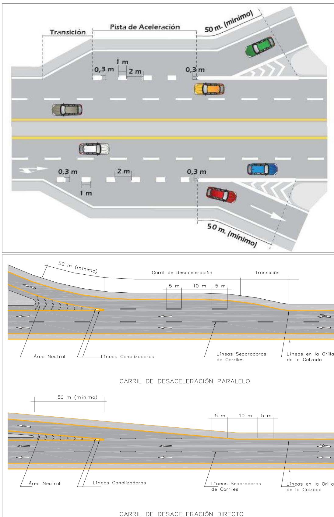
Figura 3.12 Ejemplos de líneas demarcadoras de entradas y salidas
