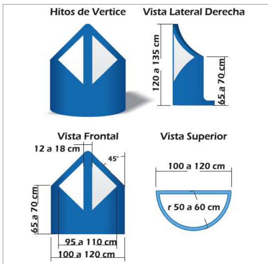
Figura 3.68 Ejemplo de dimensiones del delineador tipo “Hito de Vértice” en sus diferentes vistas
