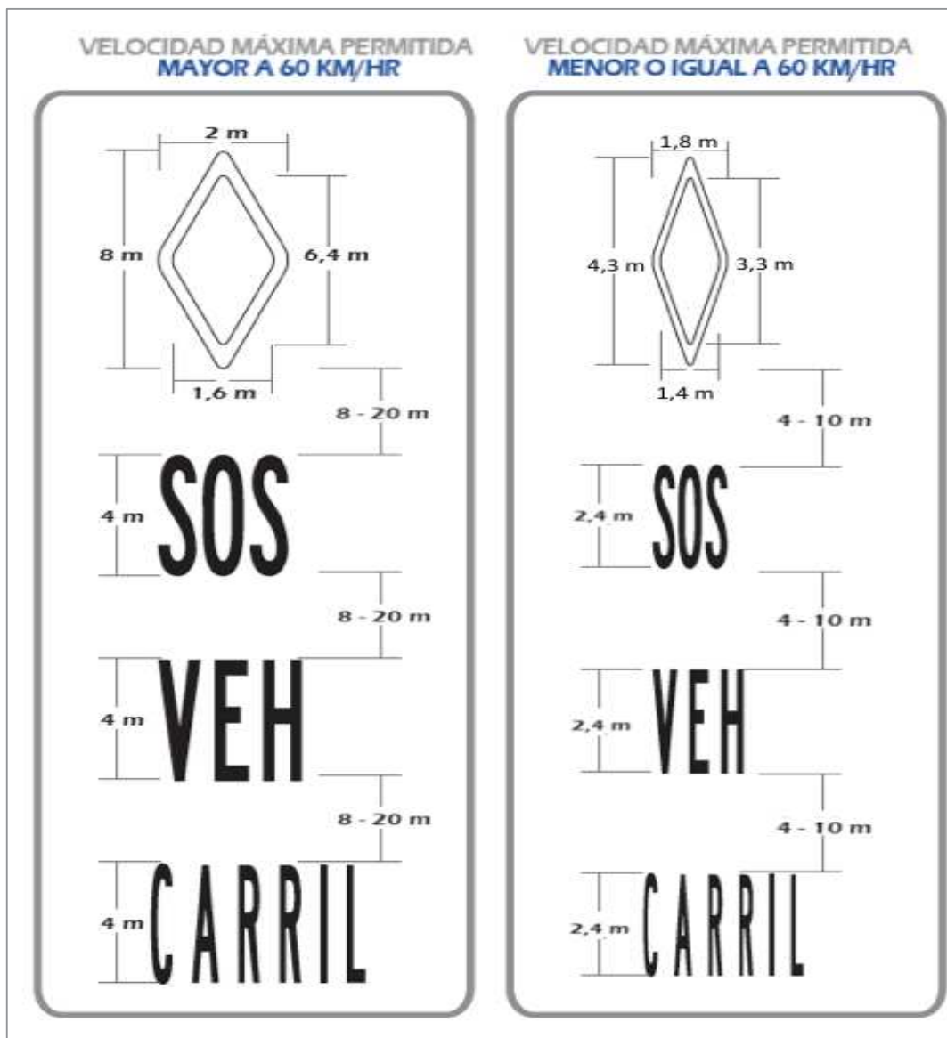
(Continúa) Figura 3.42 Ejemplo de demarcación en el pavimento de palabras, símbolos y leyendas
