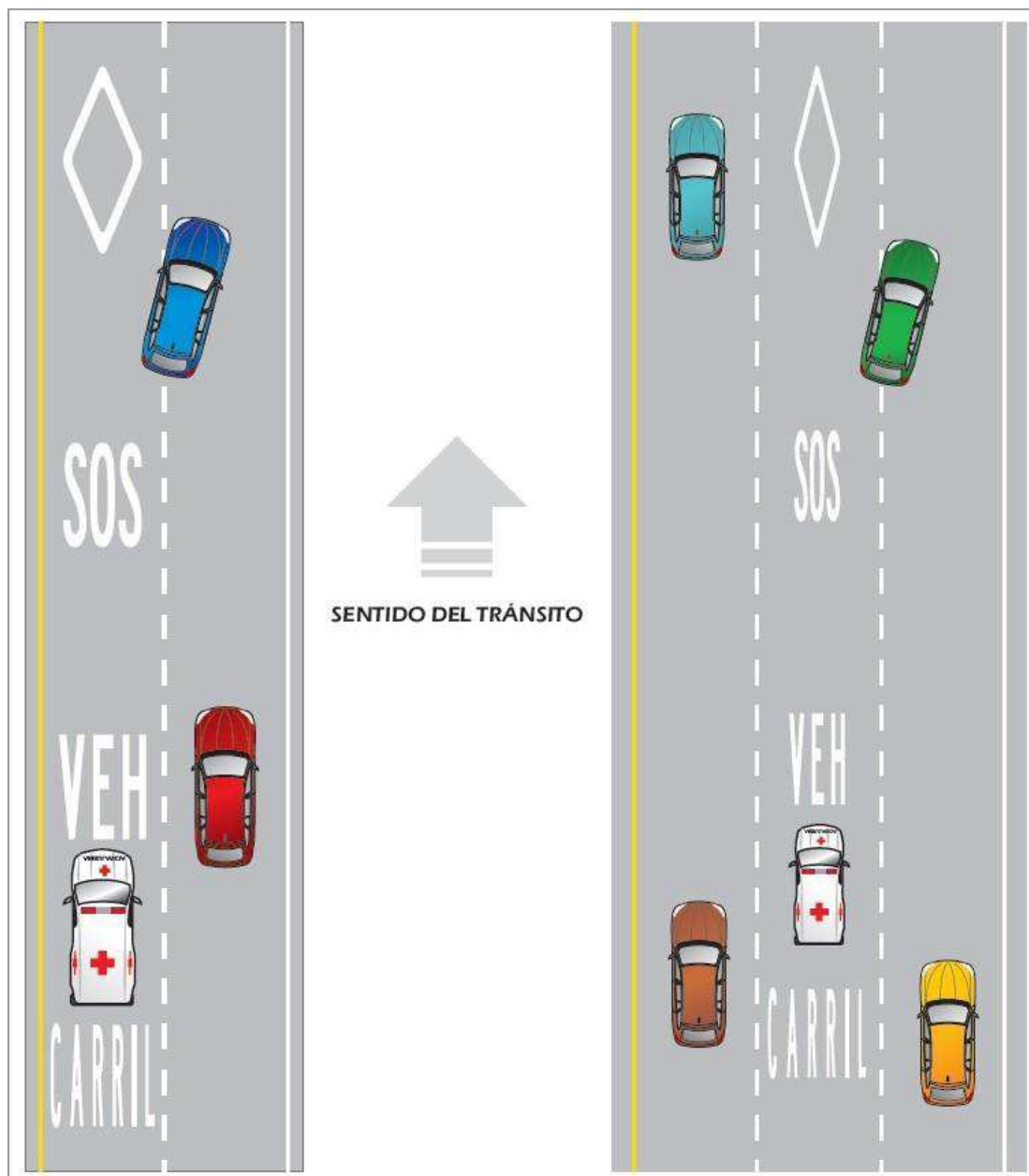
Figura 3.42 Ejemplo de demarcación en el pavimento de palabras, símbolos y leyendas
