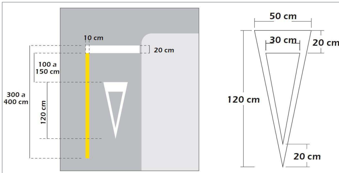
Figura 4.7 Ejemplo de dimensiones de demarcación en el pavimento "CEDA EL PASO" en intersección de "CICLOVÍA" con una vía de tránsito de vehículos motorizados.
