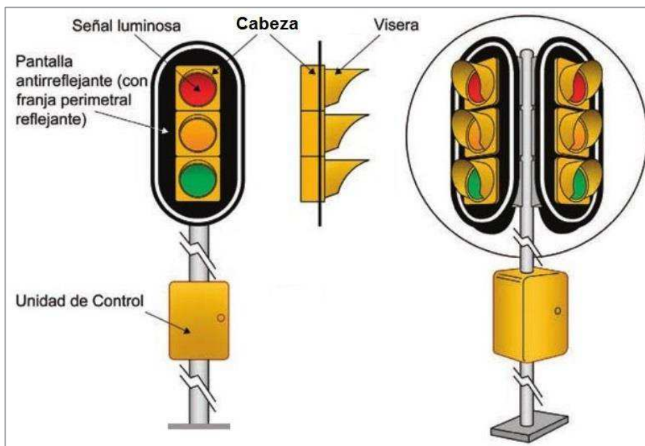
Figura 6.3 Ejemplo de configuración de cabeza de semáforos
