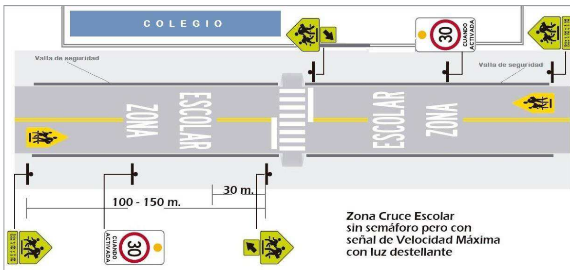
Figura 4.2 Ejemplo de señalización vertical y horizontal de una Zona Escolar
