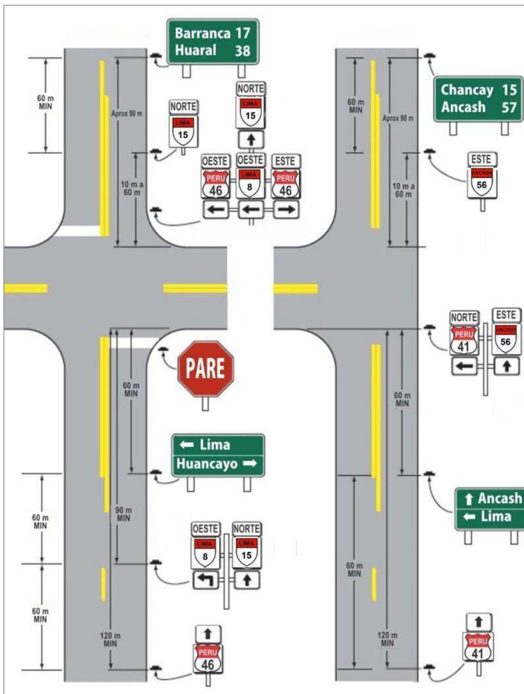
Figura 2.29 Ejemplo de conjunto de indicadores de ruta
