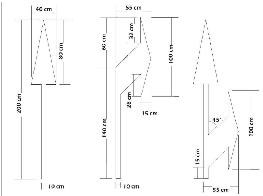
Figura 4.11 Ejemplo de dimensiones para la demarcación del símbolo tipo flecha para una “CICLOVÍA”
