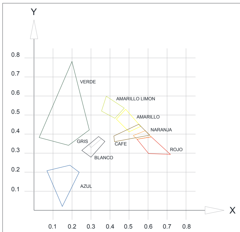
Figura 2.2 Diagrama Cromático CIE 1931
