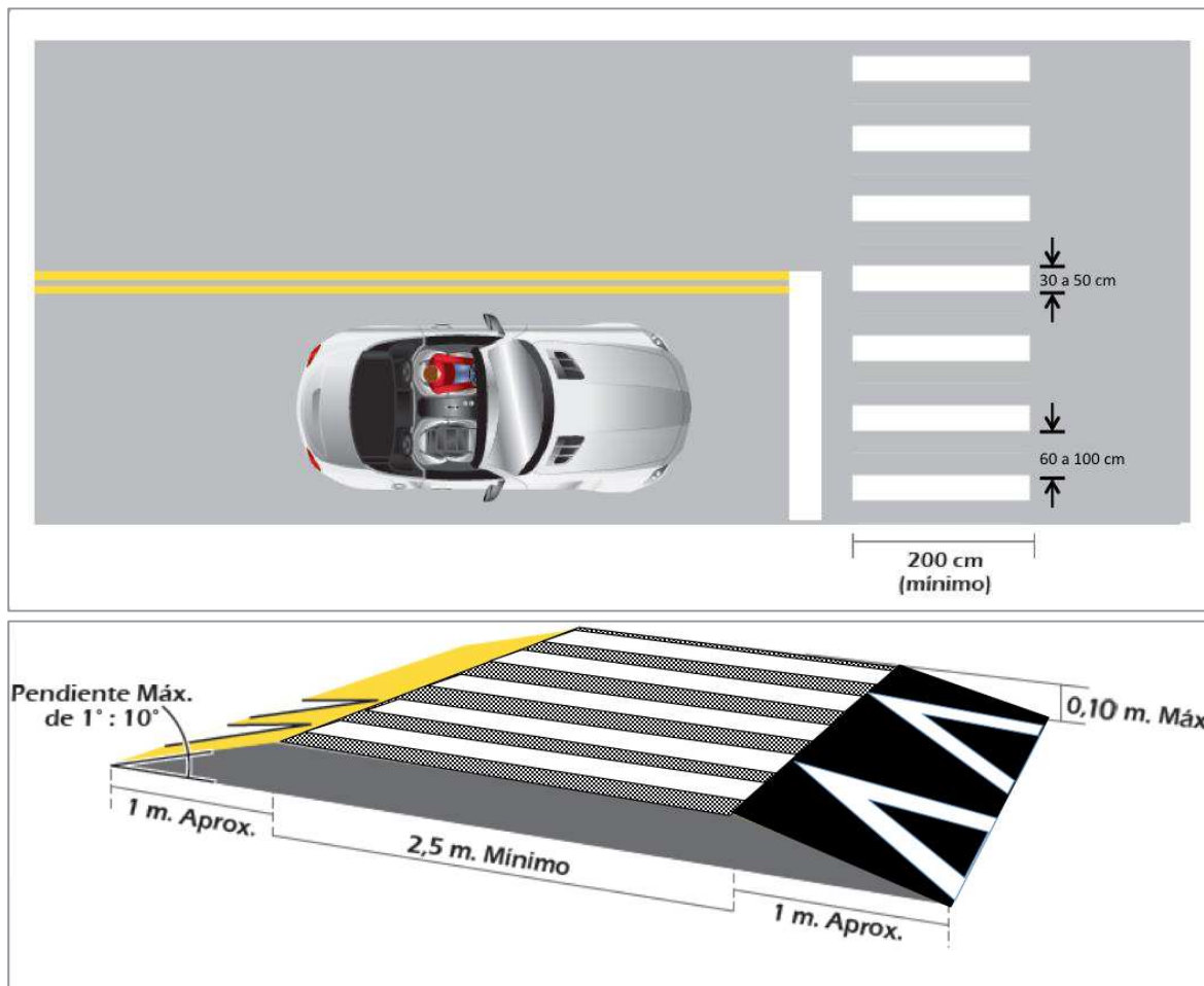
Figura 3.15 Ejemplo de demarcación líneas de cruce peatonal
