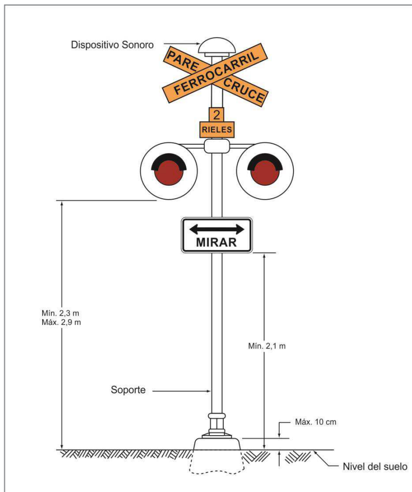
Figura 4.18 Ejemplo de un cruce peatonal a nivel con una vía férrea
