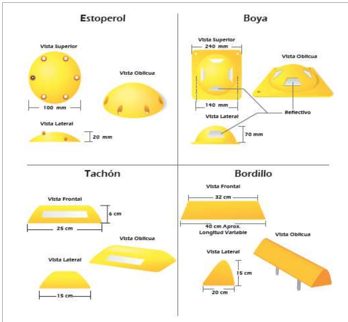
Figura 3.55 Ejemplos de otros delineadores de piso
