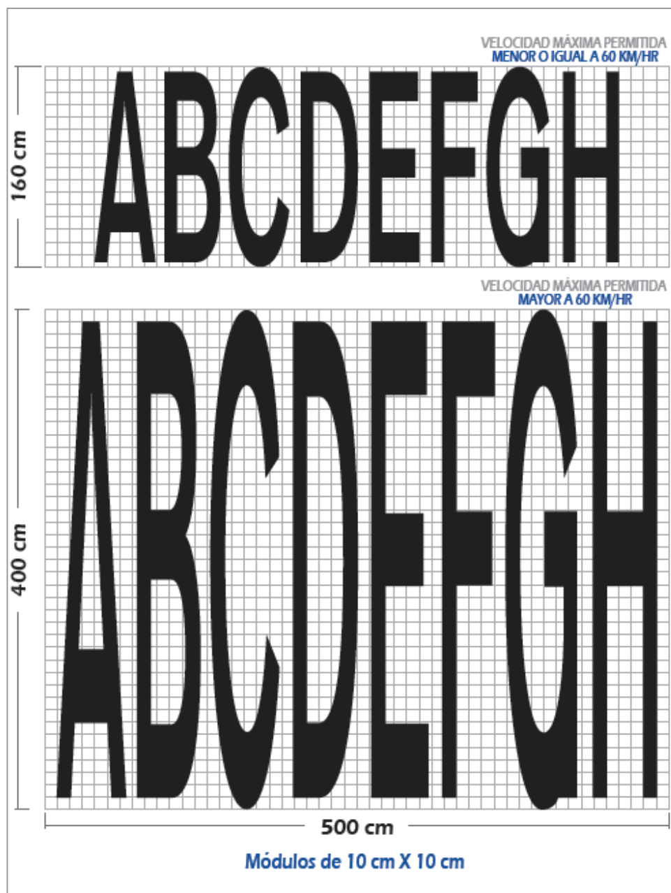
Figura 3.53 Dimensiones de la demarcación de leyenda
