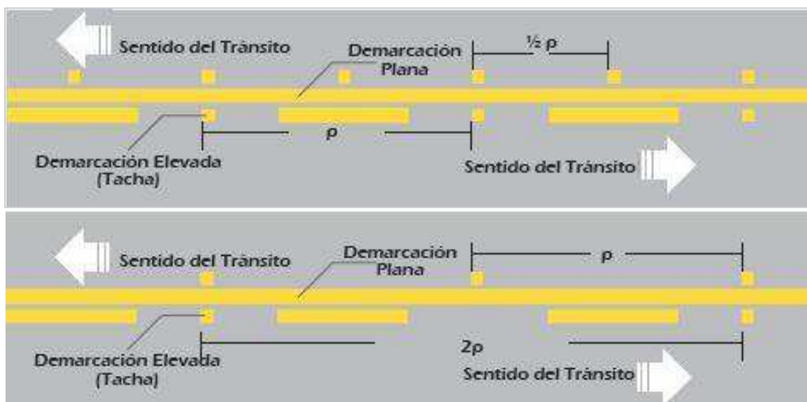
Figura 3.7 Ejemplo de líneas combinadas o mixtas
