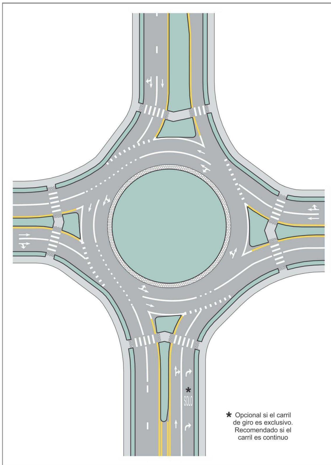
Figura 3.27 Ejemplo de demarcación para intersecciones tipo Rotonda o Glorieta de dos carriles con doble giro a la derecha
