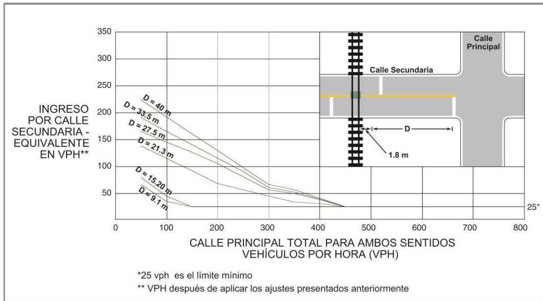
Figura 6.20 Ejemplo de condiciones de implementación semafórica en intersecciones a nivel a paso cercanos a nivel ferroviario
