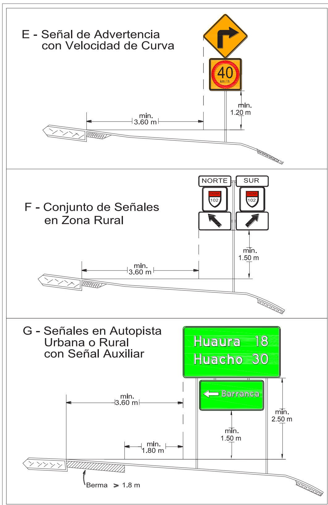
(Continua) Figura 2.5 Ejemplo de Ubicación Lateral
