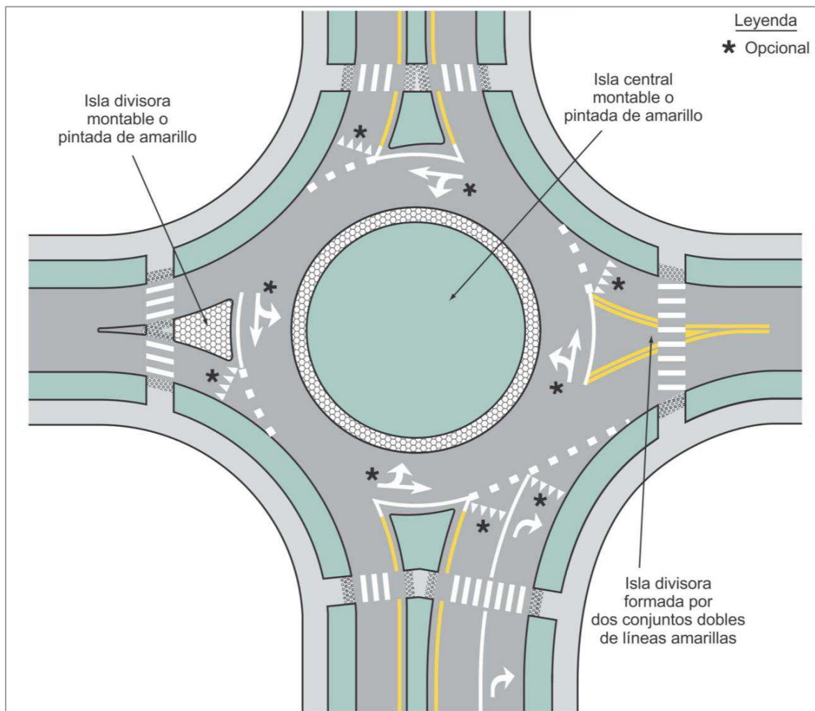
Figura 3.21 Ejemplo de demarcación para intersecciones tipo Rotonda o Glorieta de un carril
