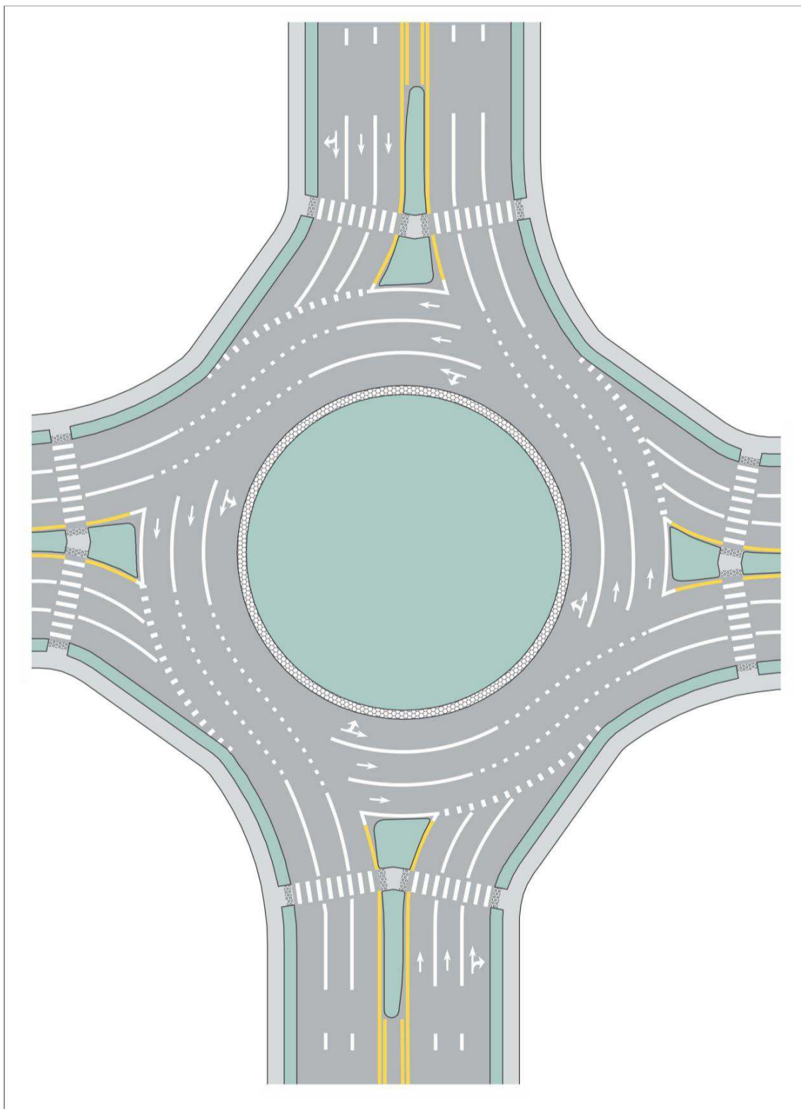
Figura 3.30 Ejemplo de demarcación para intersecciones tipo Rotonda o Glorieta de tres carriles con tres carriles de acceso
