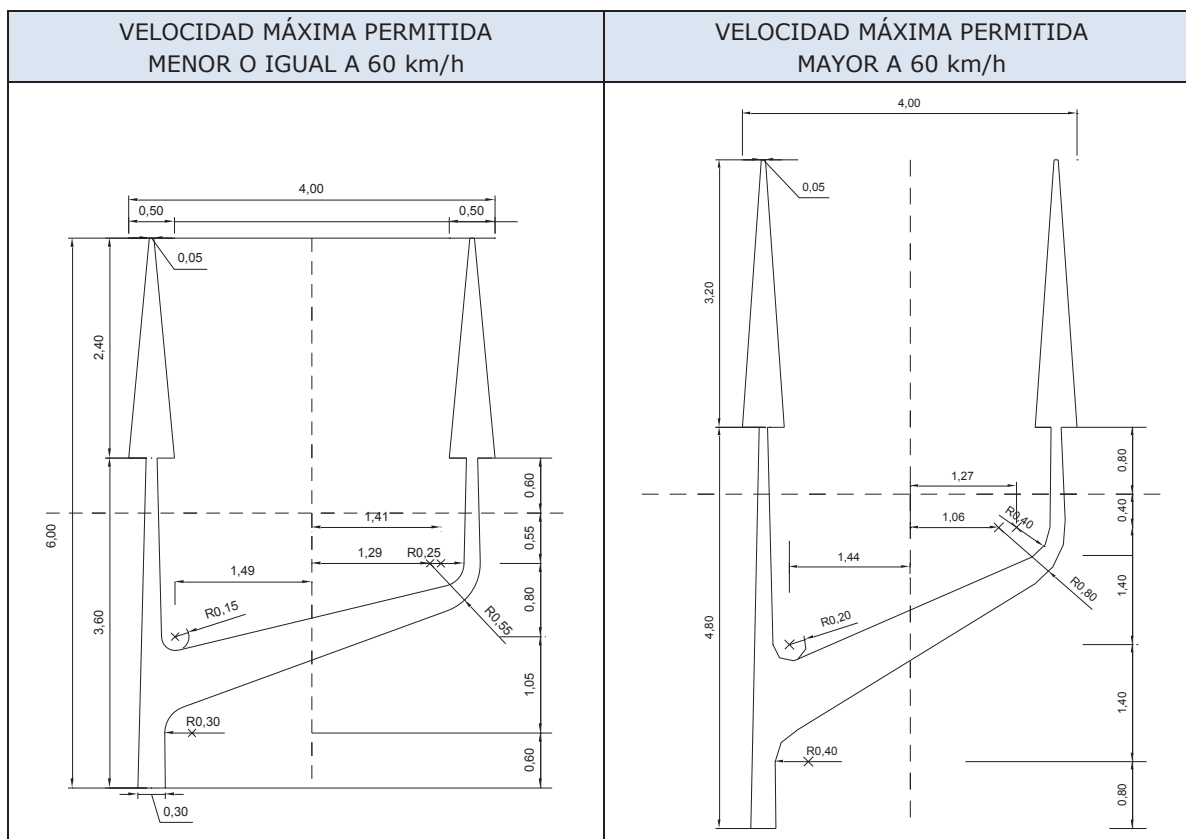
Figura 3.51 Dimensiones de flecha incorporación a carriles exclusivos
