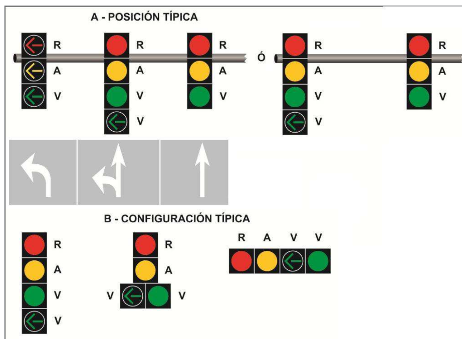
Figura 6.28 Ejemplos de disposición de indicadores de semáforos con giros a la izquierda protegidos con carril exclusivo de giro izquierda
