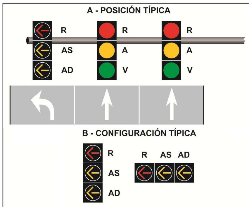
Figura 6.27 Ejemplo de disposición especial de indicadores de semáforos con giros a la izquierda permitidos (protegidos) con ámbar destellante
