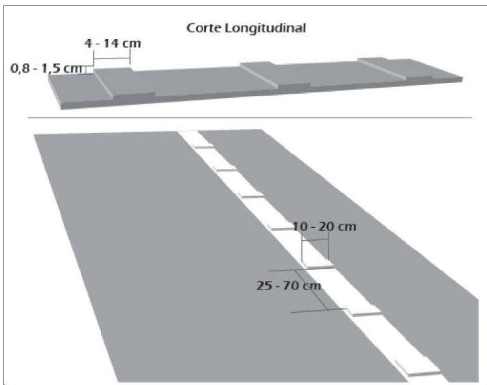
Figura 3.56 Ejemplo de demarcación resaltada
