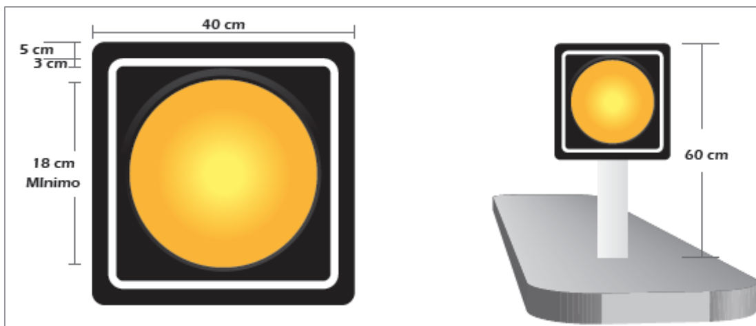
Figura 3.70 Ejemplo y dimensiones de delineadores con luces
