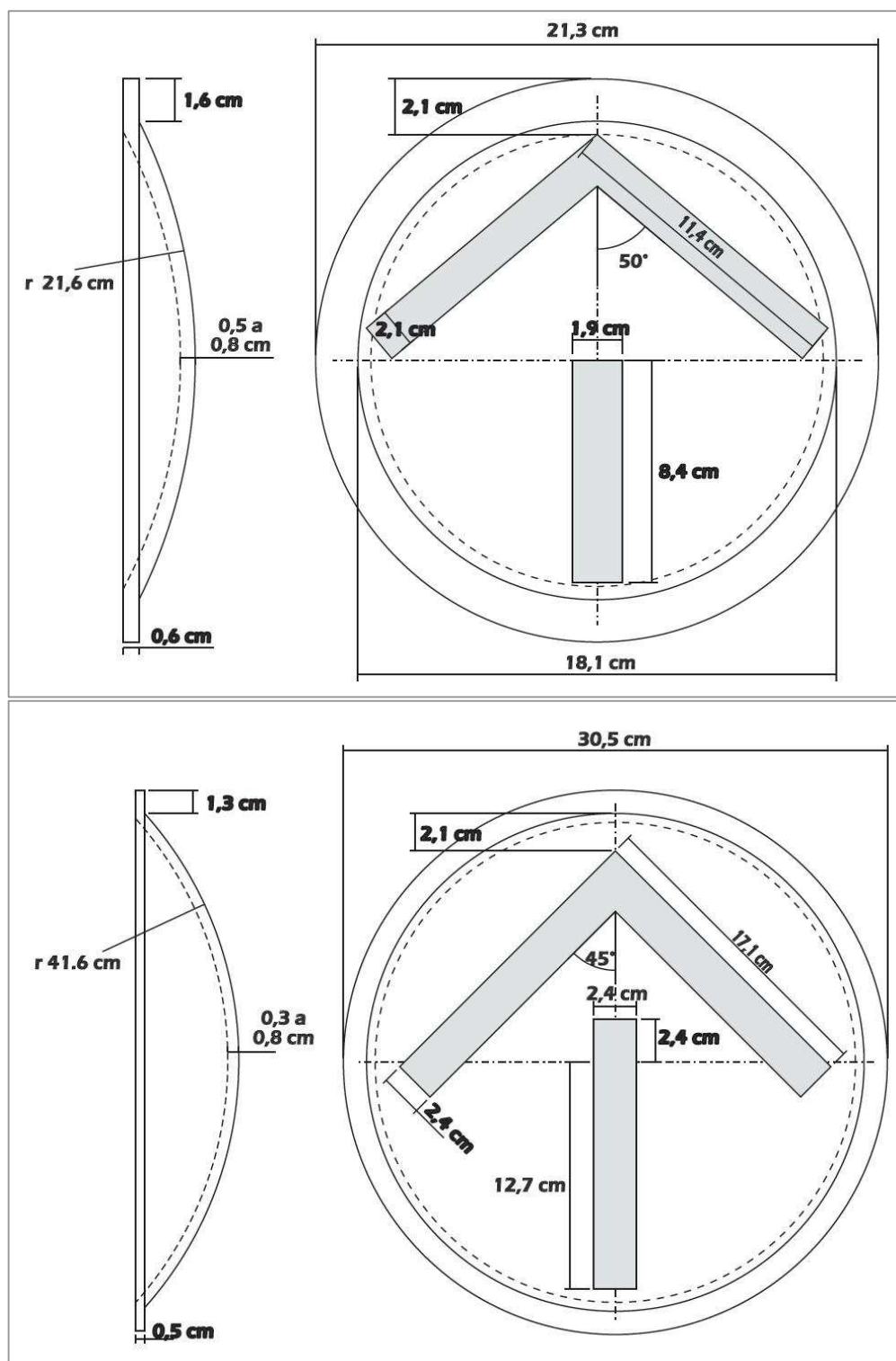
Figura 6.9 Ejemplo de lentes de 0.20 y 0.30 m
