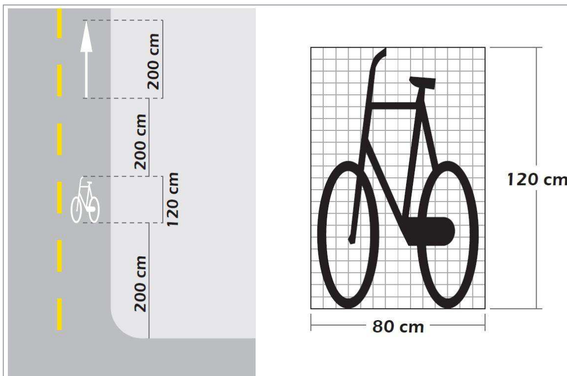
Figura 4.10 Ejemplo de demarcación en el pavimento, de las dimensiones del símbolo de una bicicleta tipo para una "CICLOVÍA"
