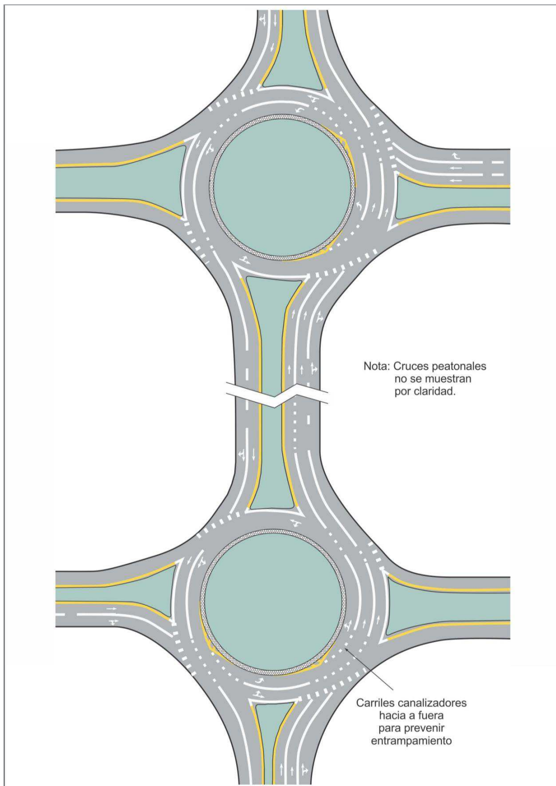
Figura 3.32 Ejemplo de demarcación para intersecciones tipo para dos Rotondas o Glorietas vinculadas
