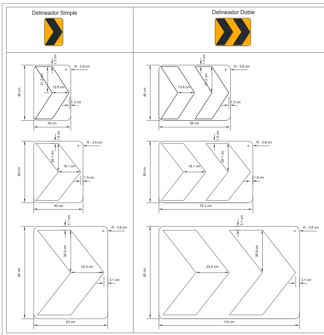
Figura 3.62 Dimensiones de los delineadores simples y dobles, en función a la velocidad máxima permitida en la vía
