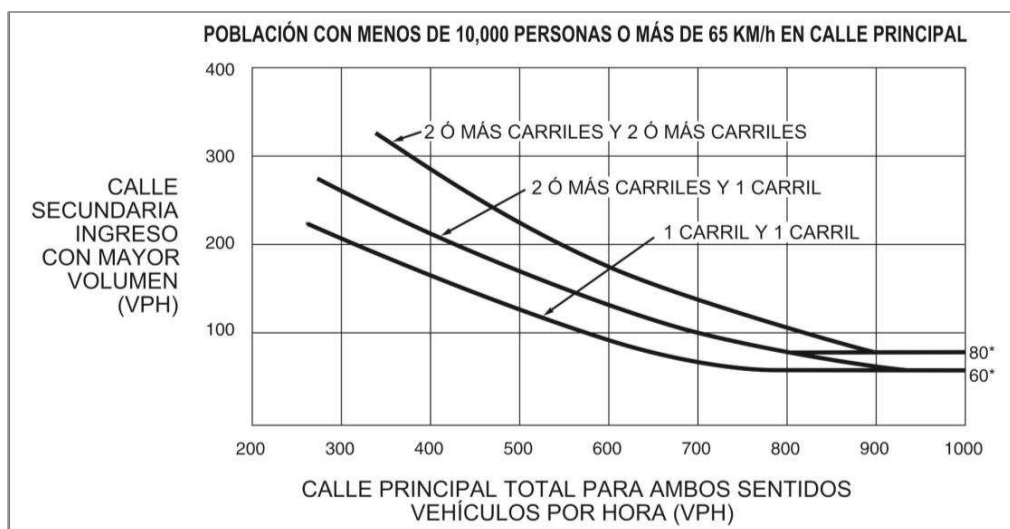
Figura 6.17: Se utiliza en función a la velocidad de la vía principal y población en zona urbana
