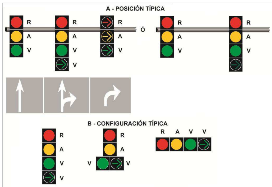
Figura 6.32 Ejemplo de disposición de indicadores de semáforos con giros a la derecha protegidos sin carril de giro exclusivo
