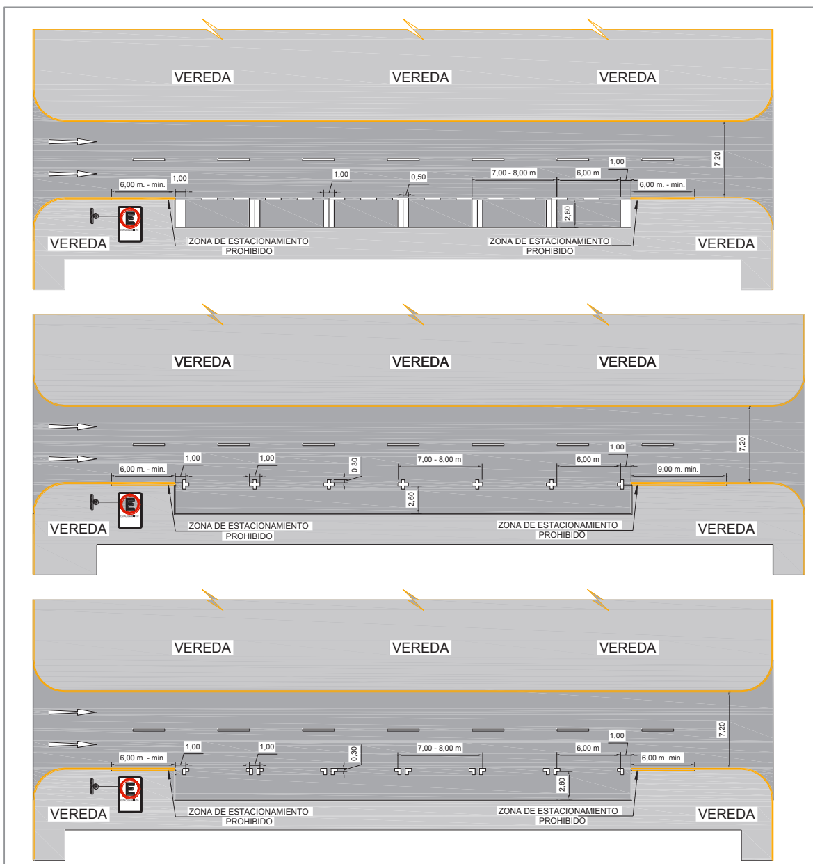
Figura 3.16 Ejemplos de demarcación en espacios para estacionamiento de vehículos con dimensiones
