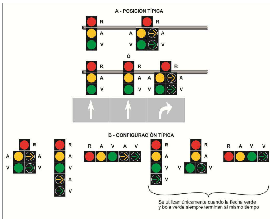
Figura 6.33 Ejemplo de disposición de indicadores de semáforos para giros a la derecha protegidos y permitidos
