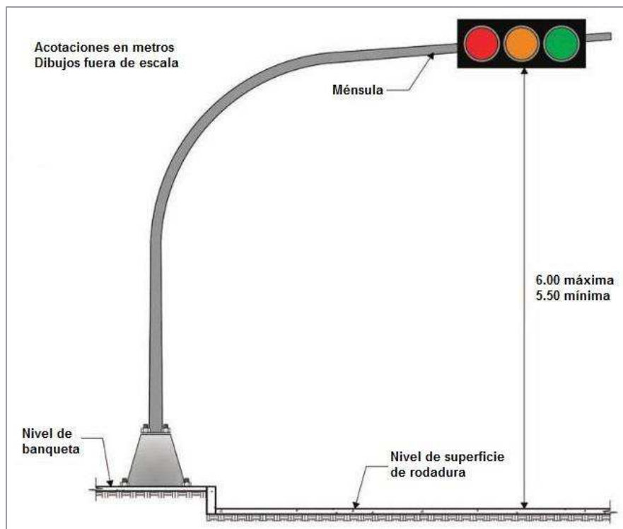
Figura 6.2 Ejemplo de soporte de semáforo tipo ménsula
