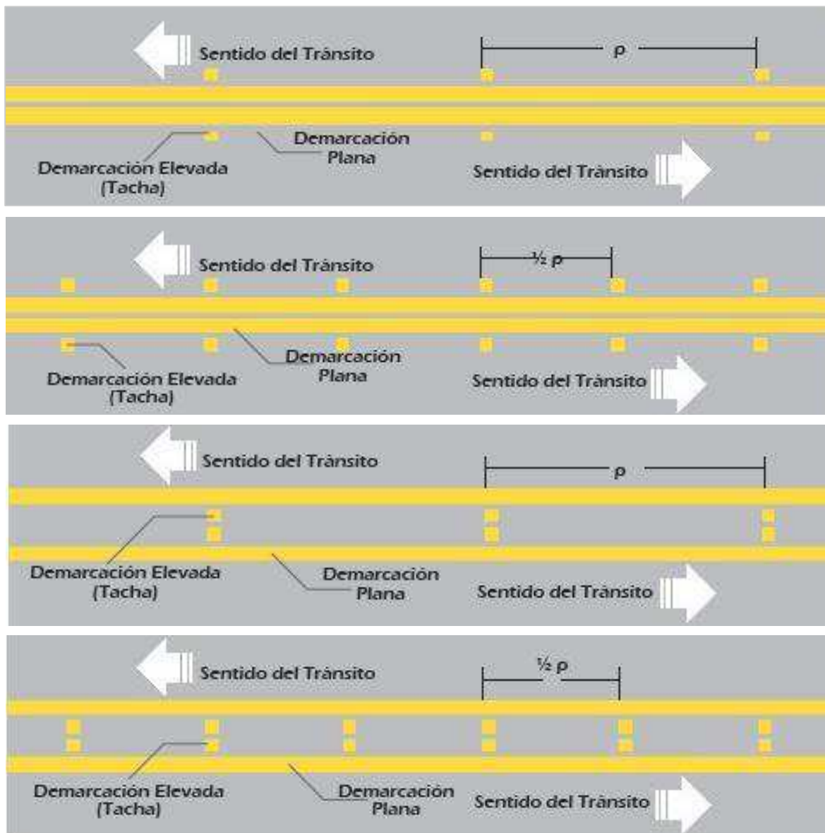
Figura 3.8 Ejemplos de línea continua doble
