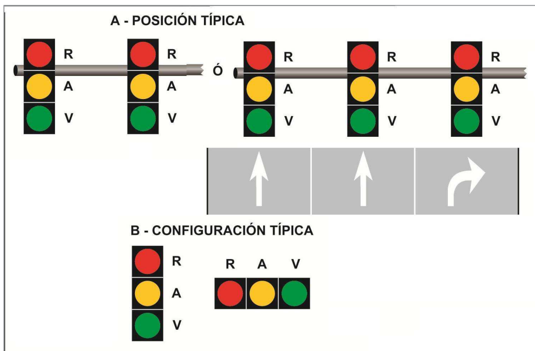
Figura 6.30 Ejemplo de disposición de indicadores de semáforos con giros a la derecha permitidos (no protegidos).
