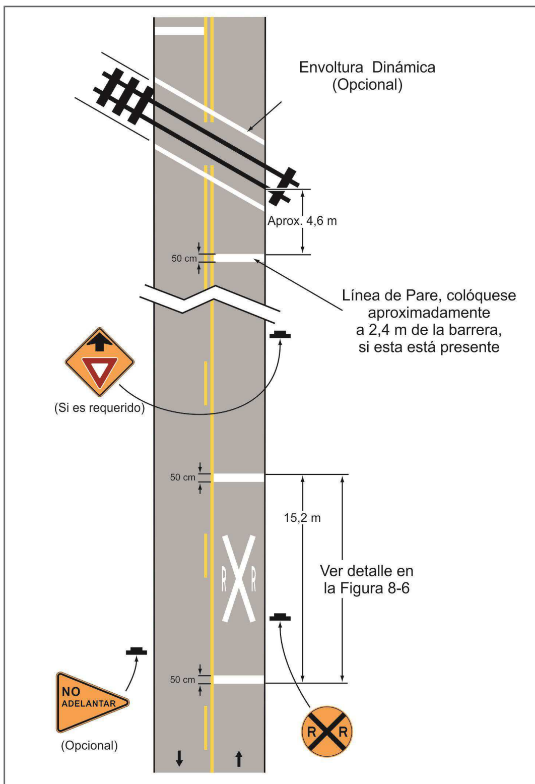
Figura 4.15 Ejemplo de señalización vertical y horizontal y dimensiones, en un cruce ferroviario a nivel oblicuo
