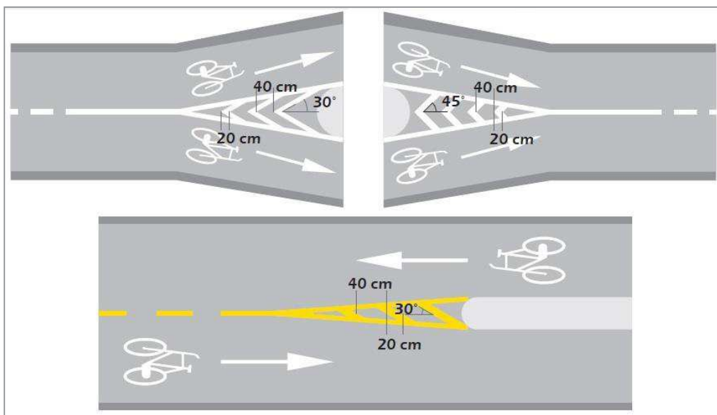
Figura 4.12 Ejemplo de demarcación de divergencias y convergencias en “CICLOVÍAS”
