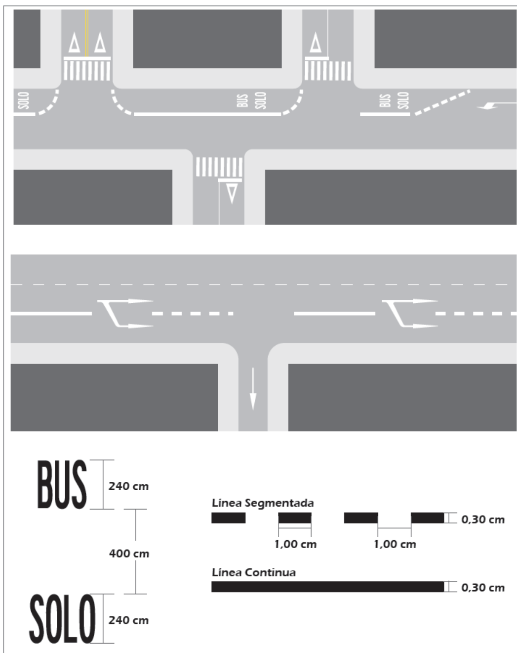
Figura 3.52 Ejemplo de aplicación de incorporación a carriles exclusivos
