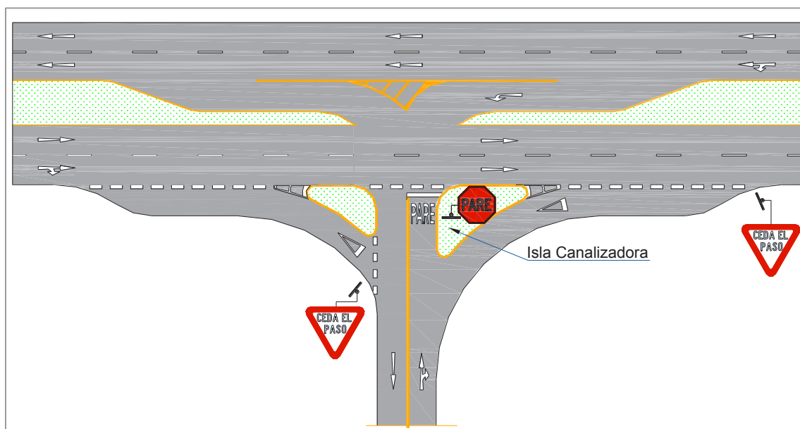
Figura 3.11 Ejemplo de demarcación en el pavimento en una intersección a nivel con islas canalizadoras
