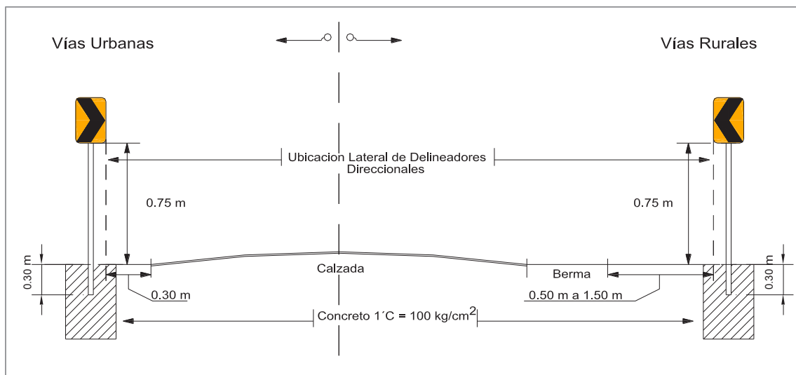
Figura 3.63 Ejemplo de ubicación de delineadores “CHEVRON”
