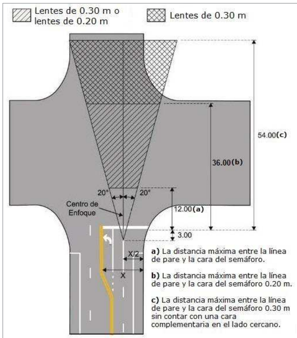
Figura 6.6 Ejemplo de ubicación de las caras de un semáforo en el lado más lejano del acceso a la intersección
