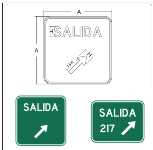
Figura 2.37 Ejemplo de señales salida inmediata
