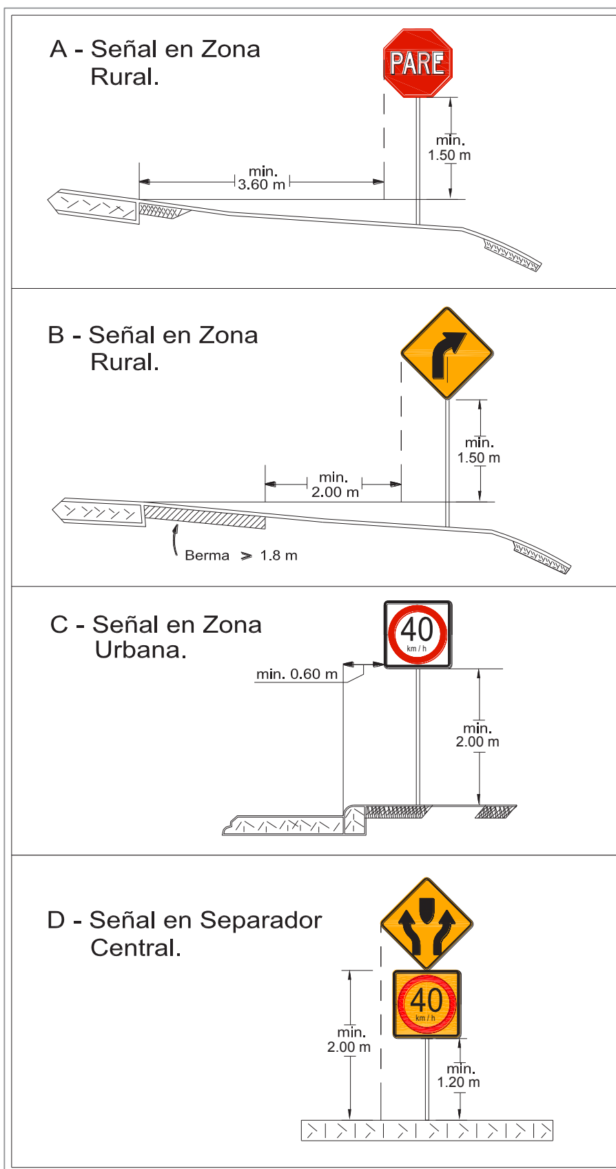
Figura 2.5 Ejemplo de Ubicación Lateral
