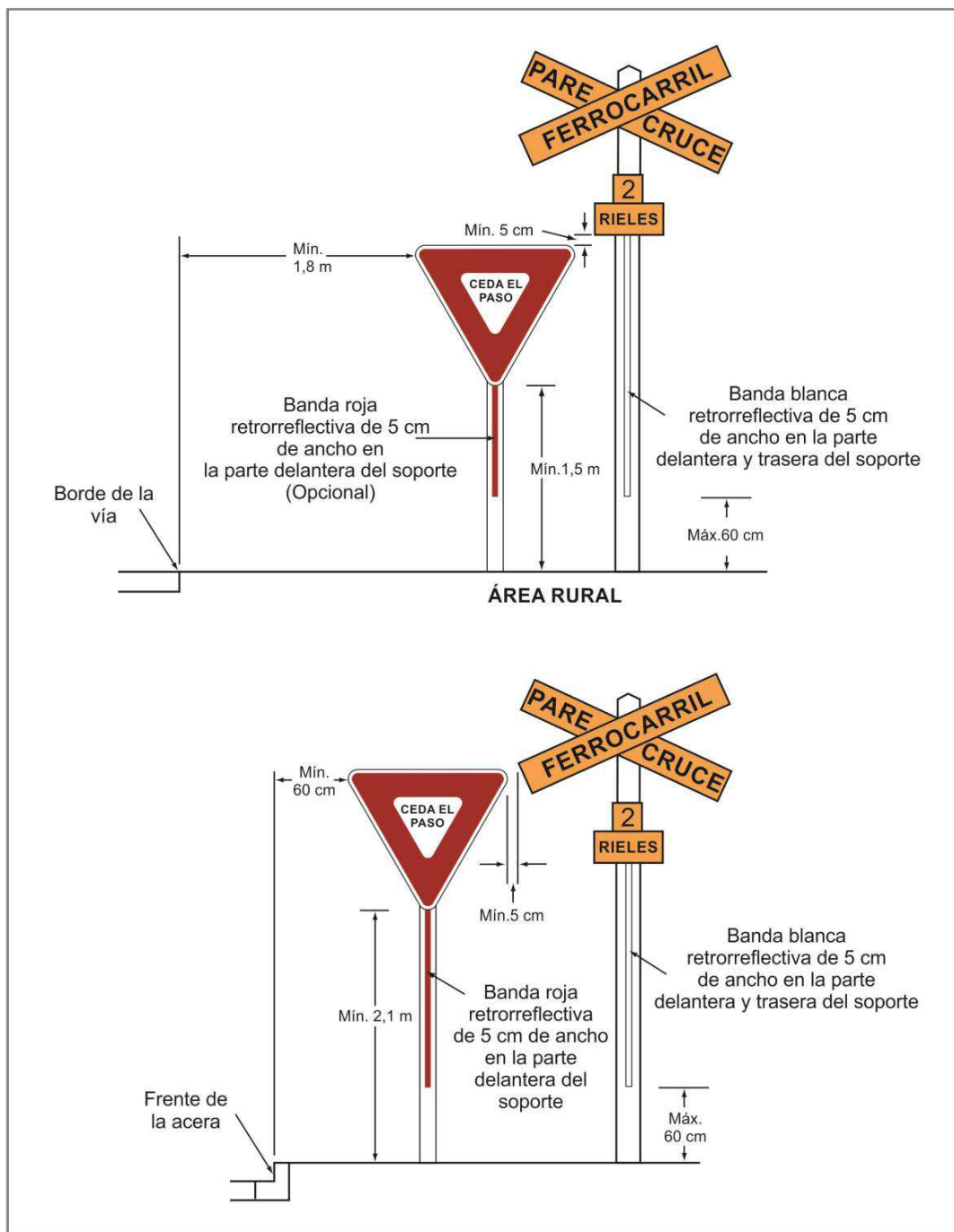
(Continua) Figura 4.14 Ejemplos de la señalización vertical y dimensiones para cruces ferroviario a nivel
