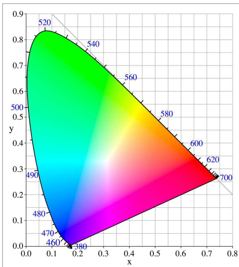
Figura 2.1 Diagrama Cromático CIE 1931
