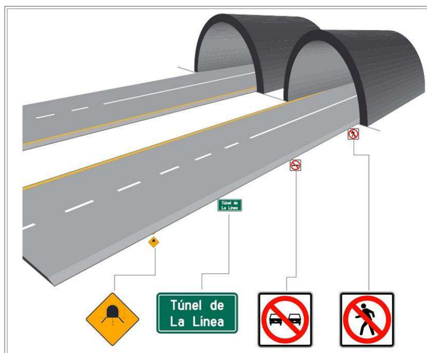
Figura 4.21 Ejemplo de señalización vertical y horizontal en la zona previa de acceso a un doble túnel o gemelos
