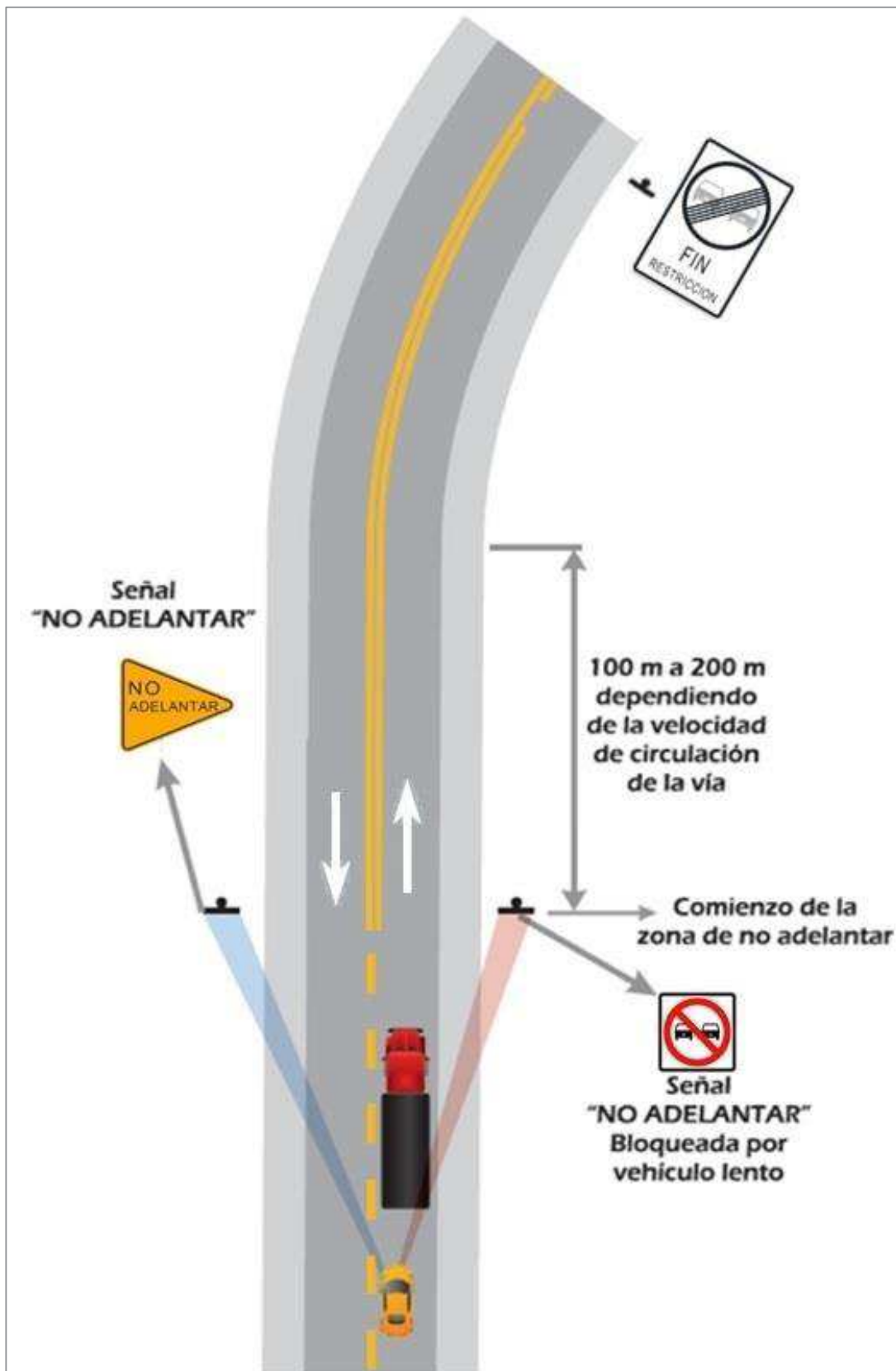
Figura 3.10 Ejemplo de zona o tramo con prohibición de adelantamiento complementado con señalización vertical
