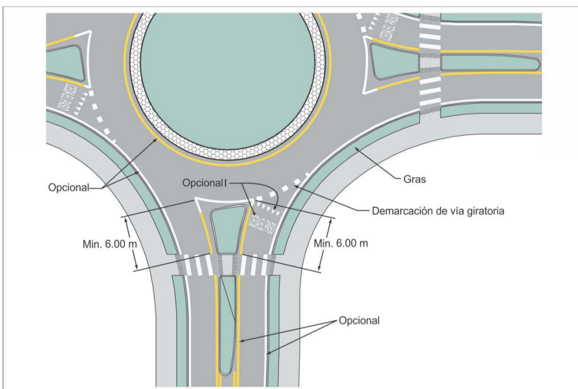
Figura 3.20 Ejemplo de demarcación para intersecciones tipo Rotonda o Glorieta en las aproximaciones de ingreso y salida, y de un carril giratorio
