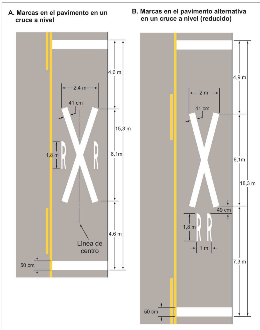
Figura 4.16 Ejemplo de demarcación en el pavimento y dimensiones de un cruce ferroviario a nivel
