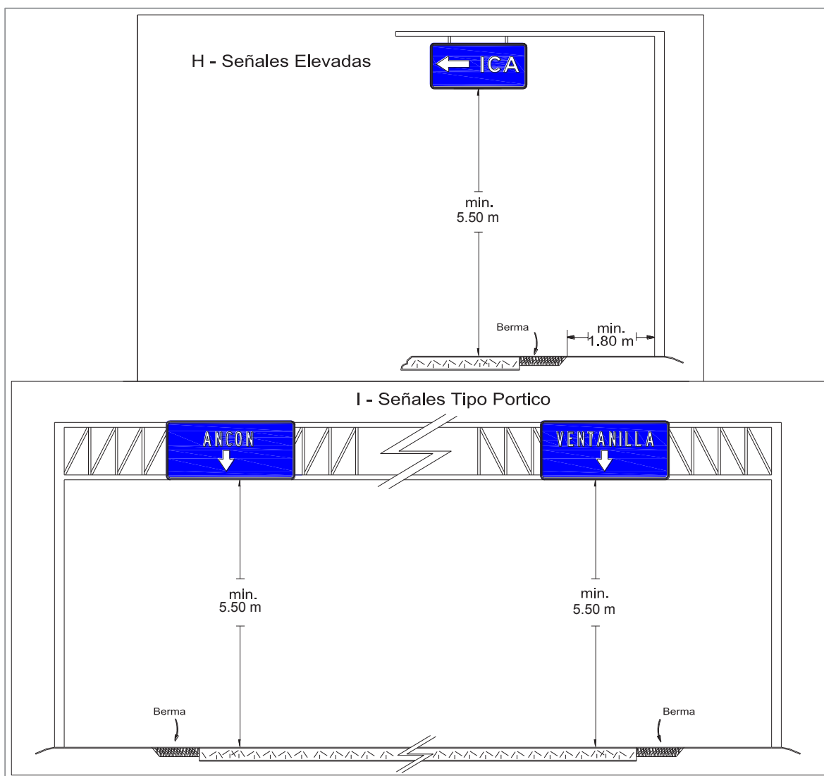
(Continua) Figura 2.5 Ejemplo de Ubicación Lateral
