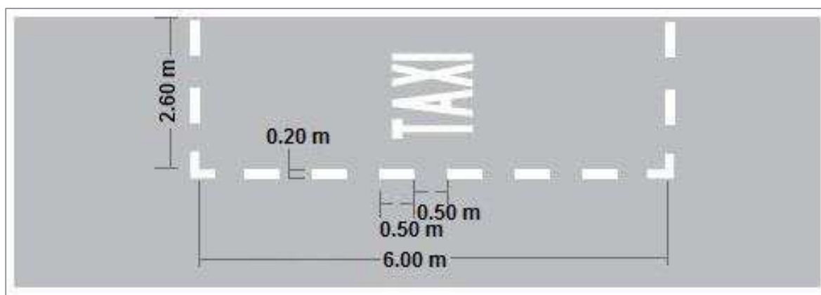
Figura 3.17 Ejemplo de demarcación de estacionamiento para servicios de taxi
