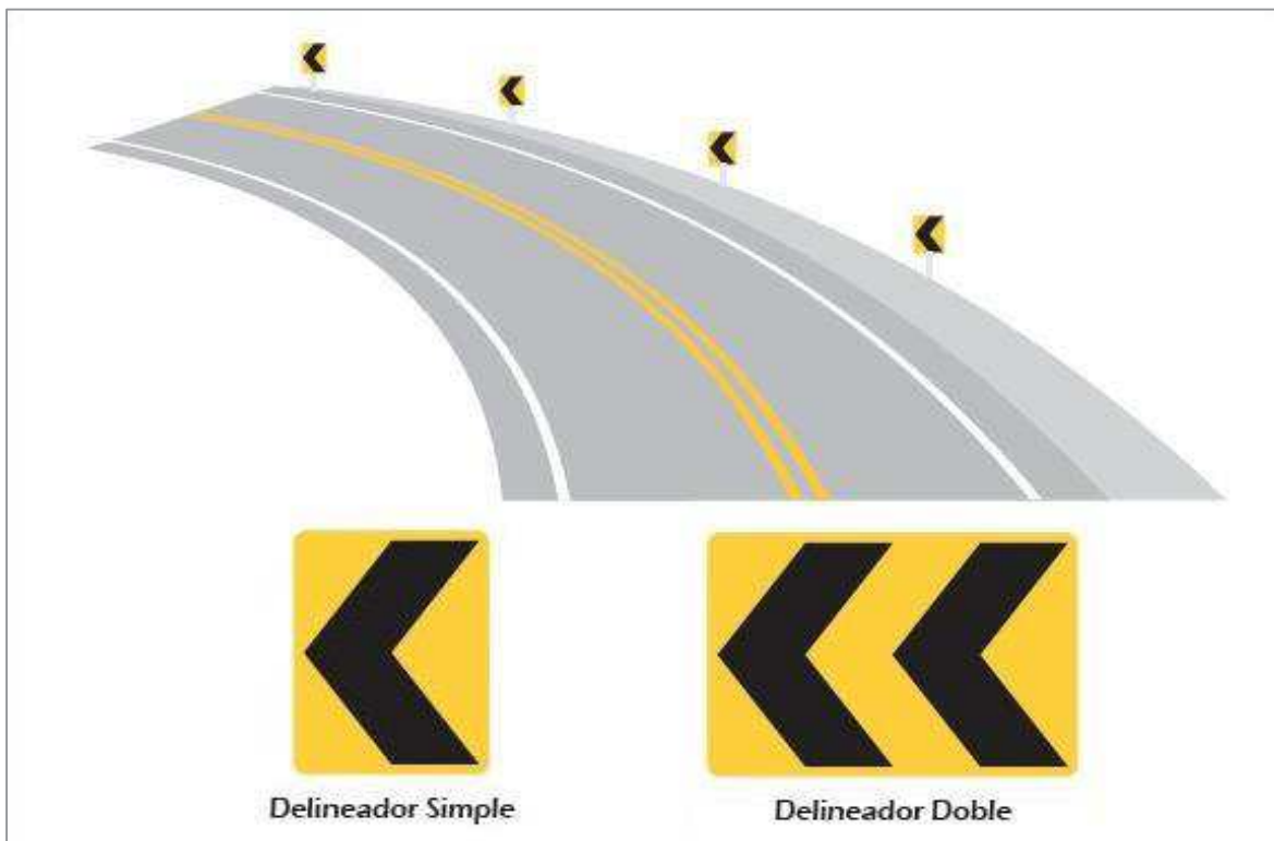
Figura 3.61 Ejemplo de señales de delineador de curva horizontal "CHEVRON"
